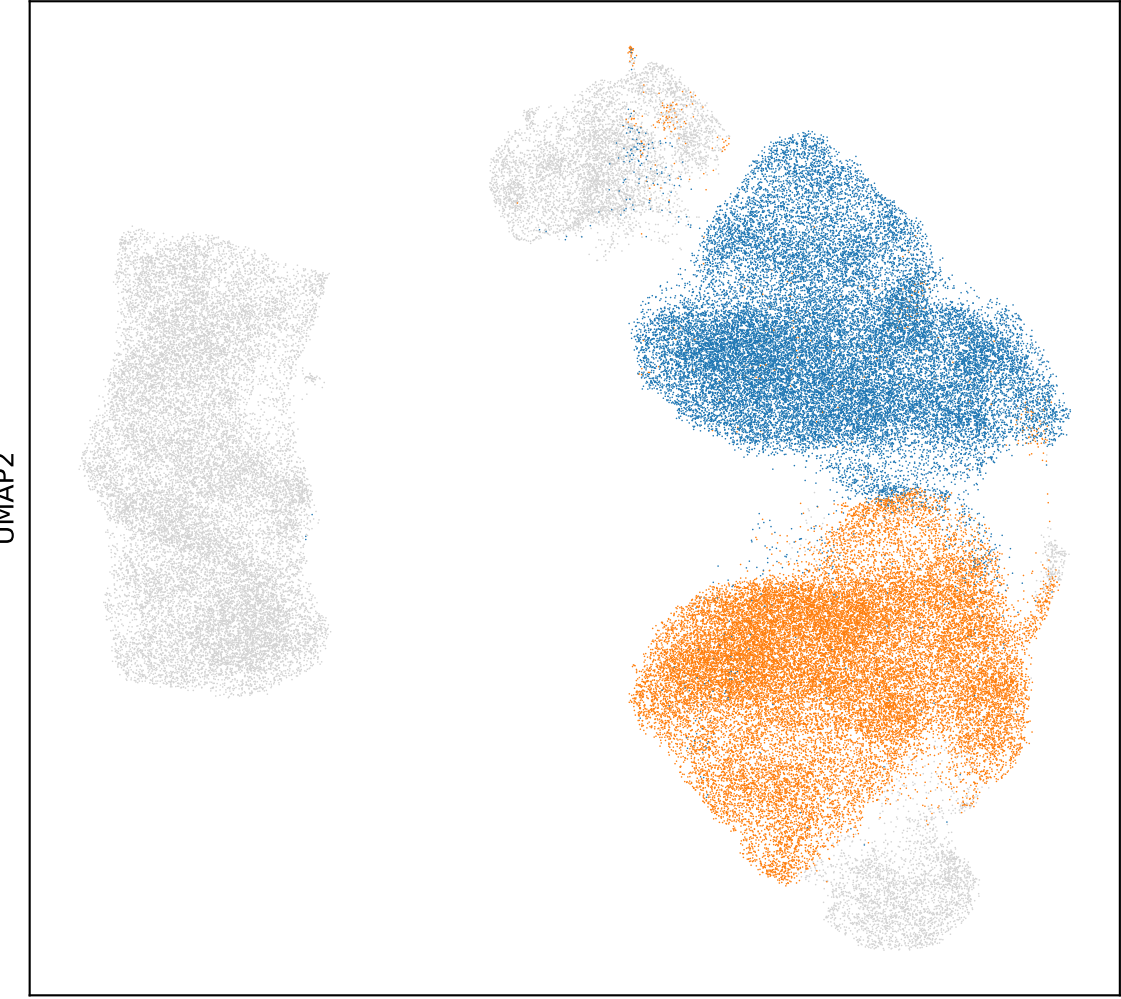
D1_vs_D2
