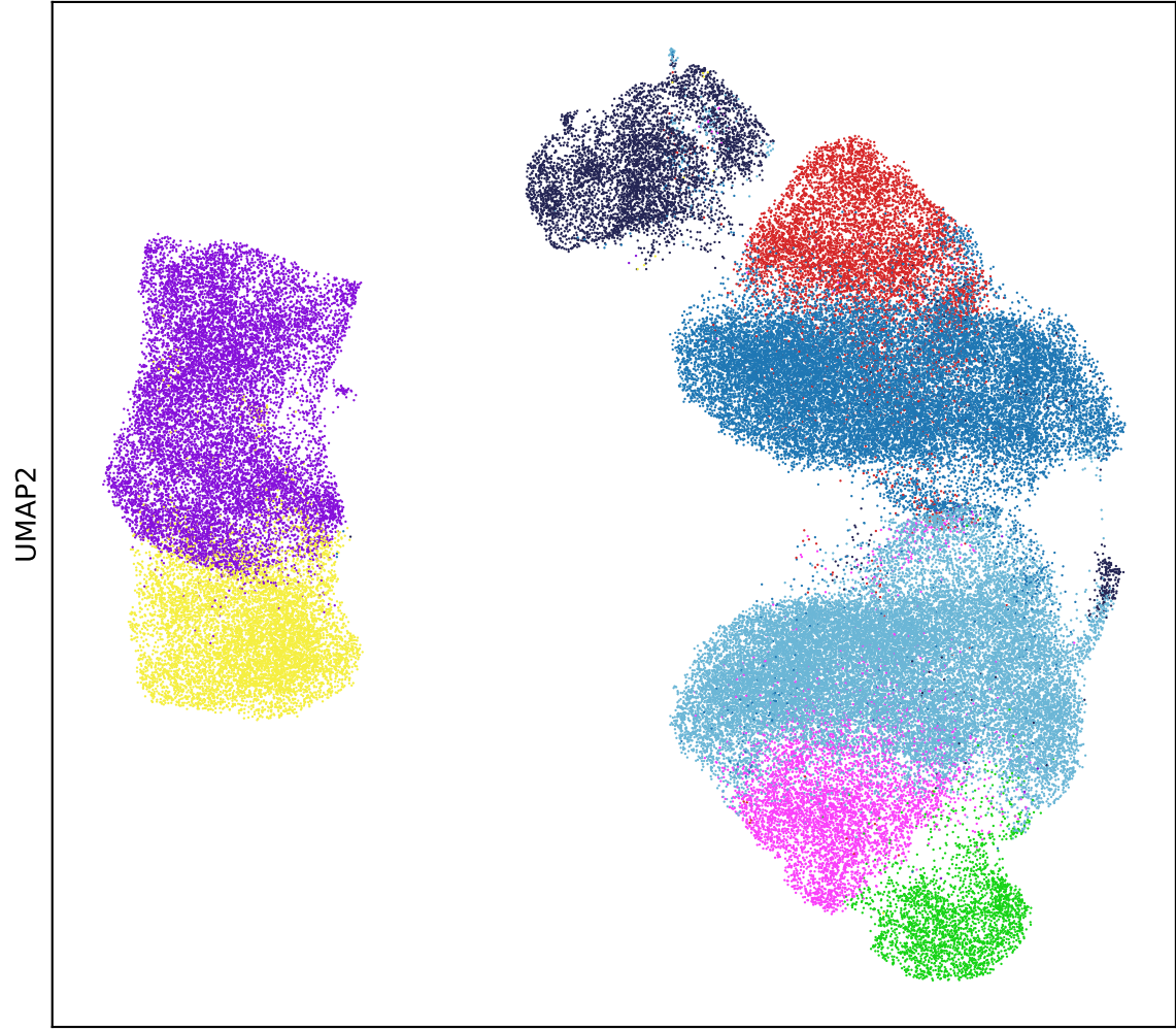
SlideTag
