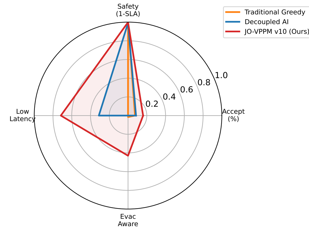
KPI Radar
