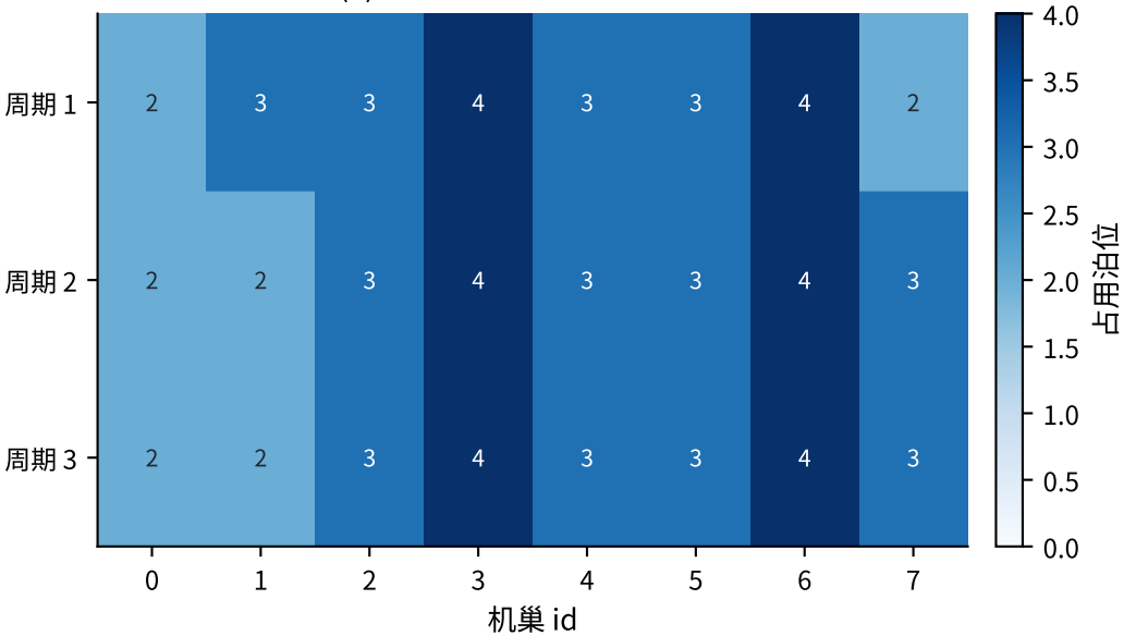
(c) 机巢泊位占用 (容量 4)
