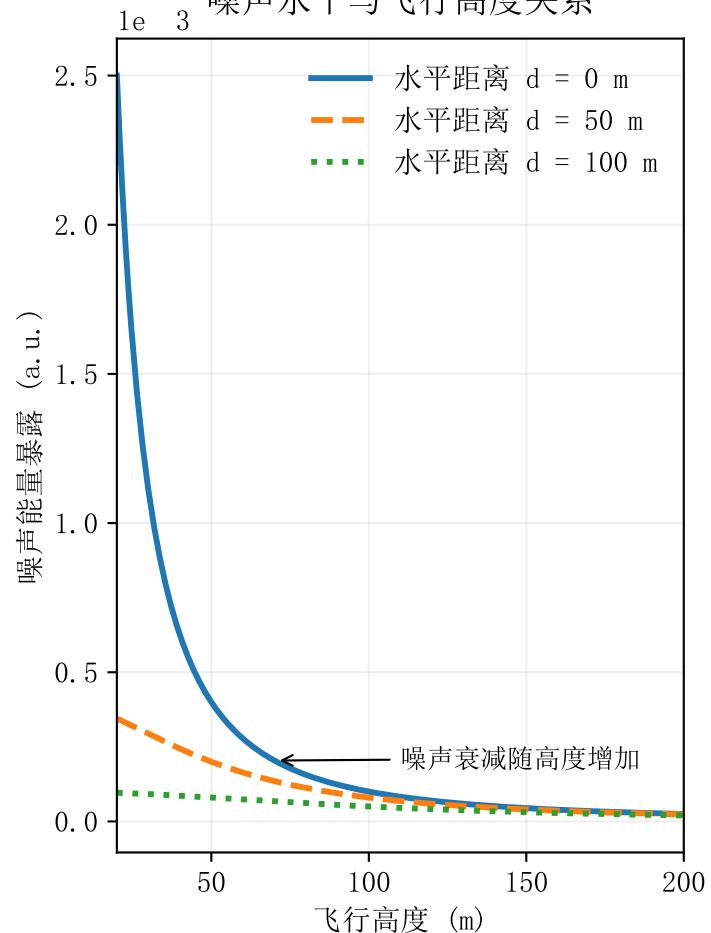
噪声水平与飞行高度关系
