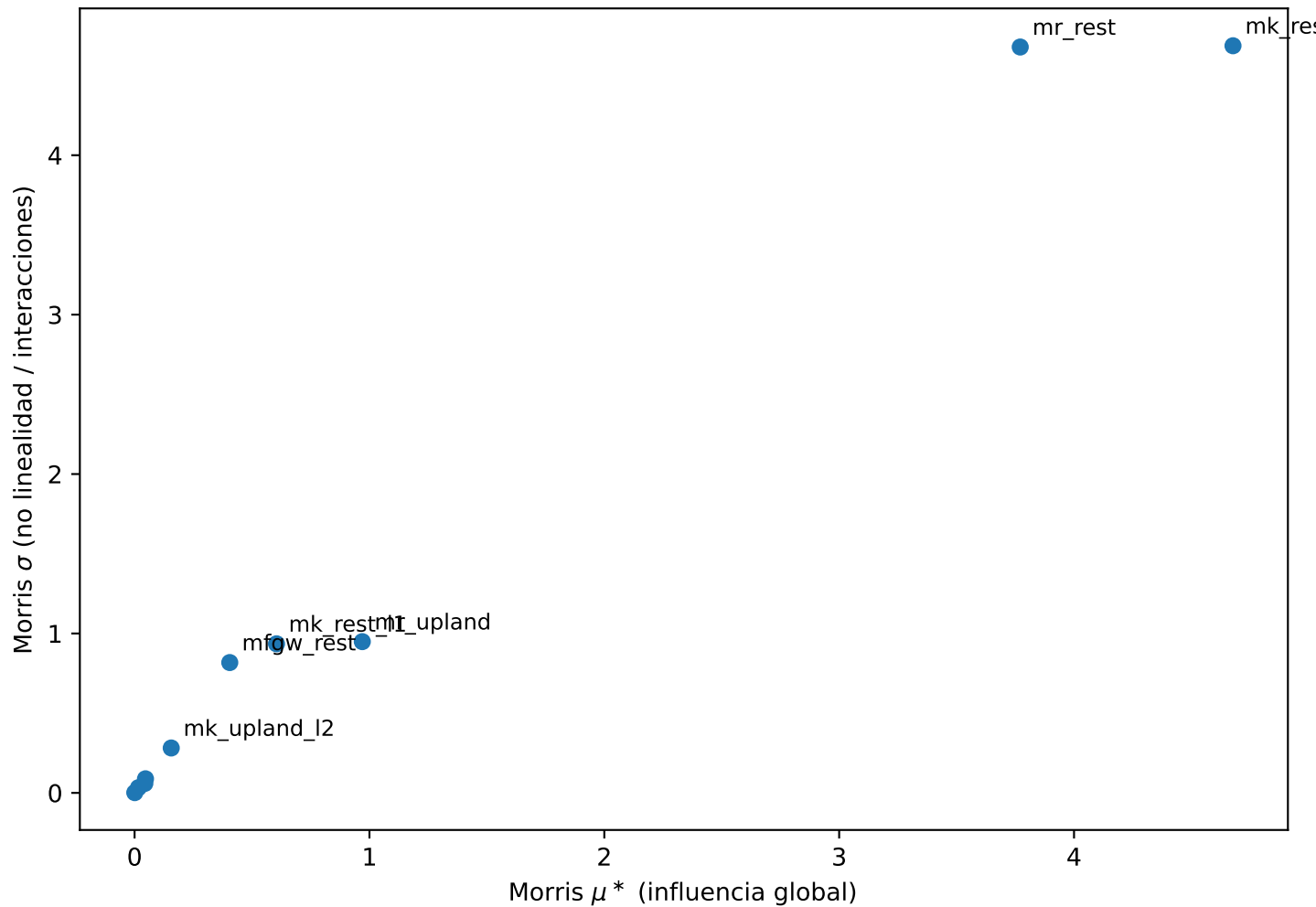
Diagrama de Morris: influencia global sobre RMSE de heads
