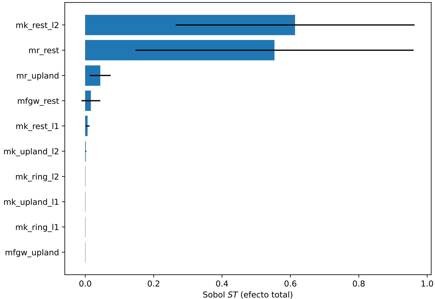
Sobol (ST): efecto total sobre RMSE de heads
