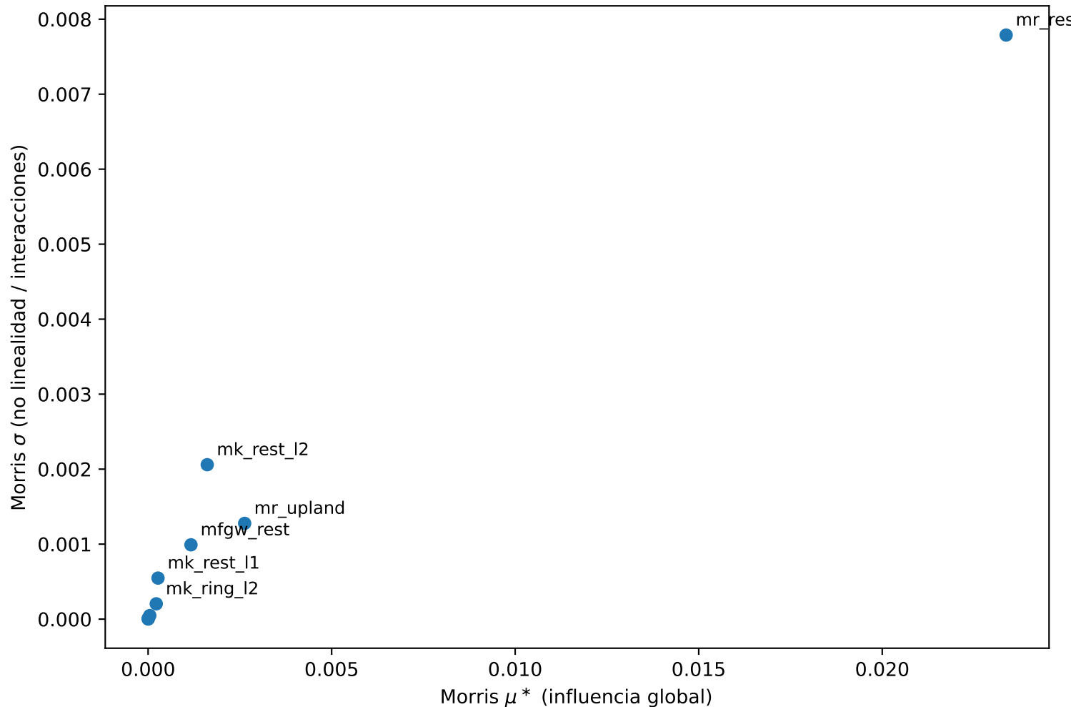
Diagrama de Morris: influencia global sobre RMSE de SGD
