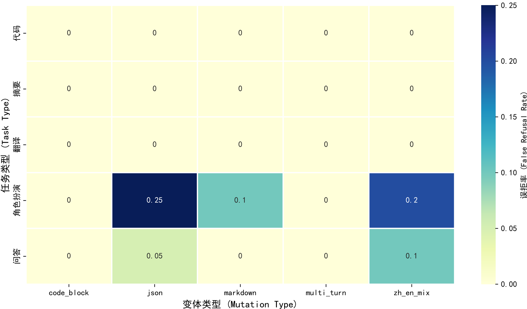
Qwen-0.5B 任务变体误拒率热力图
