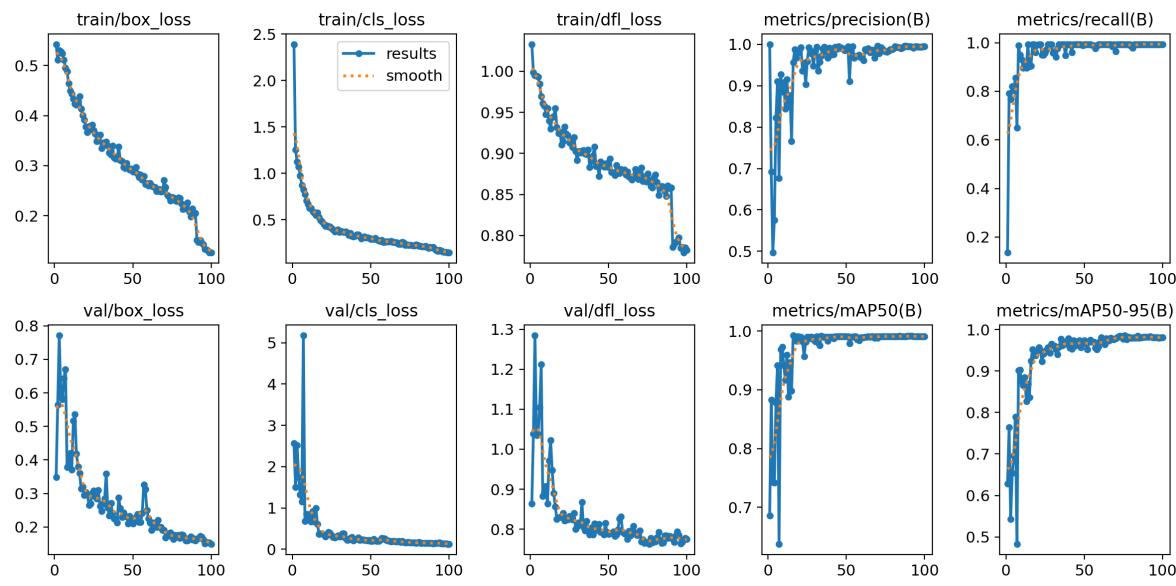
图 3. 训练过程指标曲线（仓库 results/training/results.png）
