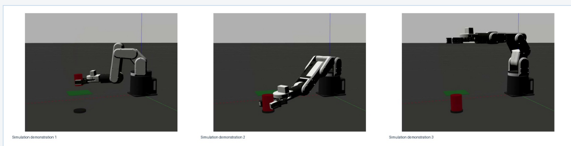
用于定点抓取与放置验证的仿真动作序列
