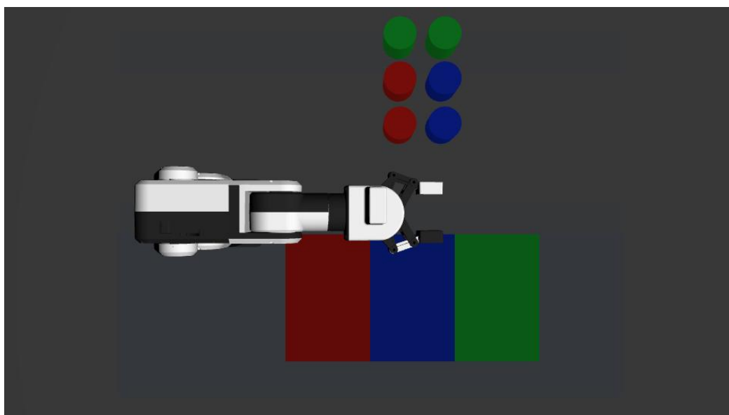
图 3 Gazebo 三分类场景：六个取物格与同排分类垫
