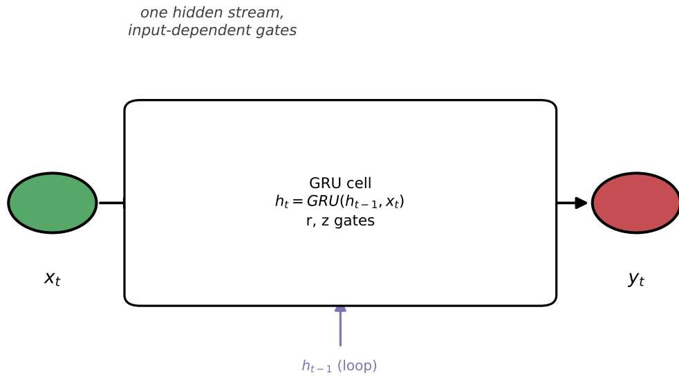
(a) GRU — baseline
