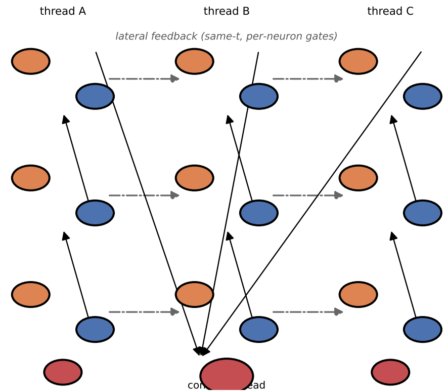
(d) MFN 3L3T — threaded grid (width of streams)
