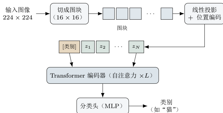
图 5.6: Vision Transformer (ViT)：图像切成固定大小的图块，每块经线性投影加位置编码成为一个视觉 token；连同一个额外的“[类别]” token 一起送入 Transformer 编码器，最后由分类头输出类别。
