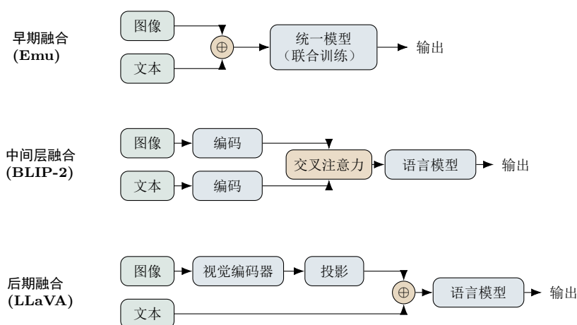
图 5.15: 三类融合按“融合发生的早晚”区分（ \oplus / 交叉注意力为融合点，由上到下依次后移）：早期融合（Emu）在输入端就把图文嵌入并入同一序列、统一建模；中间层融合（BLIP-2）各自编码后用交叉注意力在编码器与语言模型之间交互；后期融合（LLaVA）让视觉先经独立编码器完整编码，末端才与文本拼接接入语言模型。
