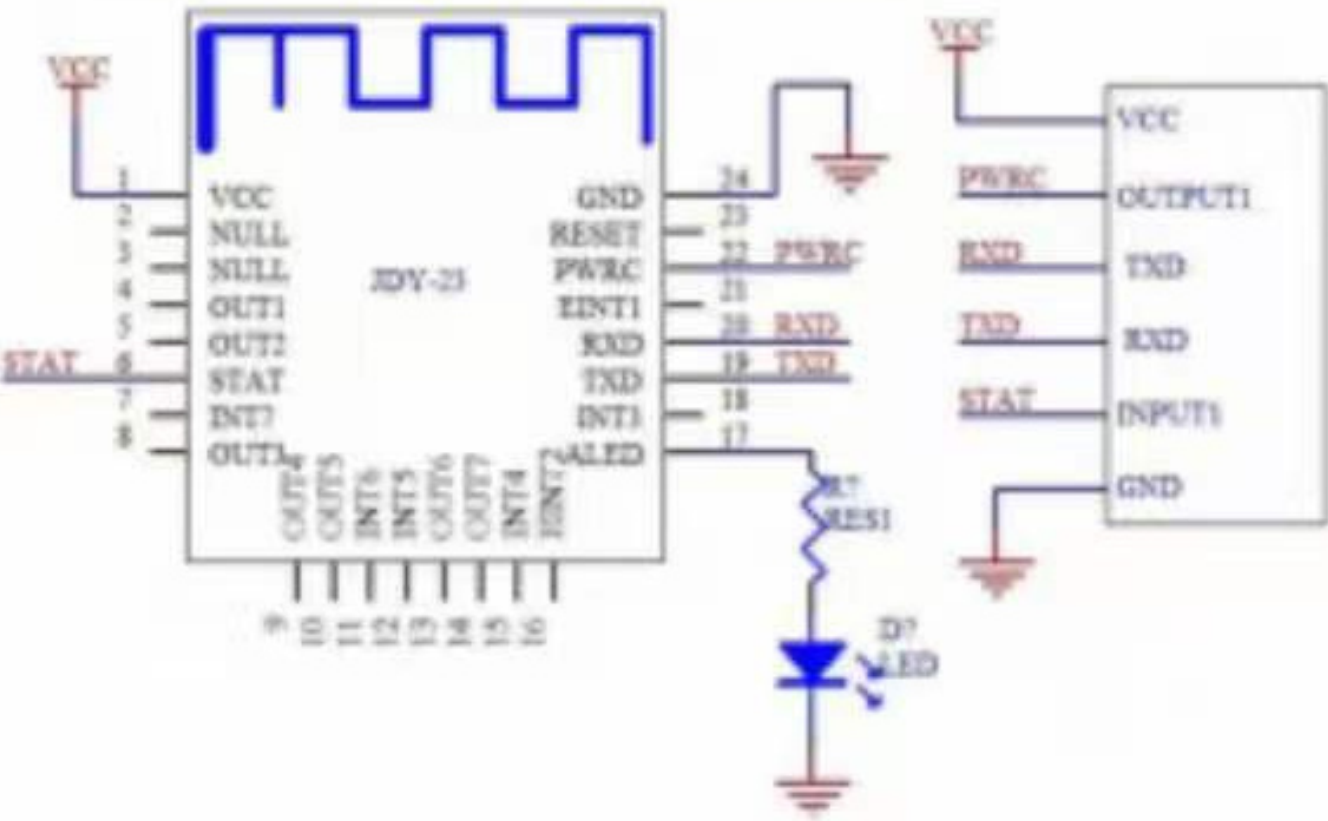
JDY-23 手机APPP控制OUT引脚高低电平与读取INT引脚电平接线图
