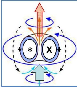
Рис.4. Эфиродинамический Торонд со Спином-Джетом в свободном эфире – схематическое обозначение.
