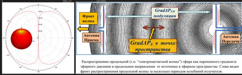
Рис.2а. Продольная неударная эфирная “Электромагнитная волна” ( V = C ).
