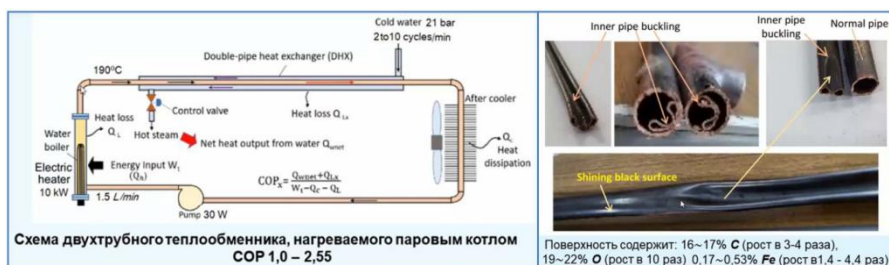
Рис. 22. Двухтрубный Кавитационный Реактор - слева. Деформация внутренней трубы реактора- справа.
