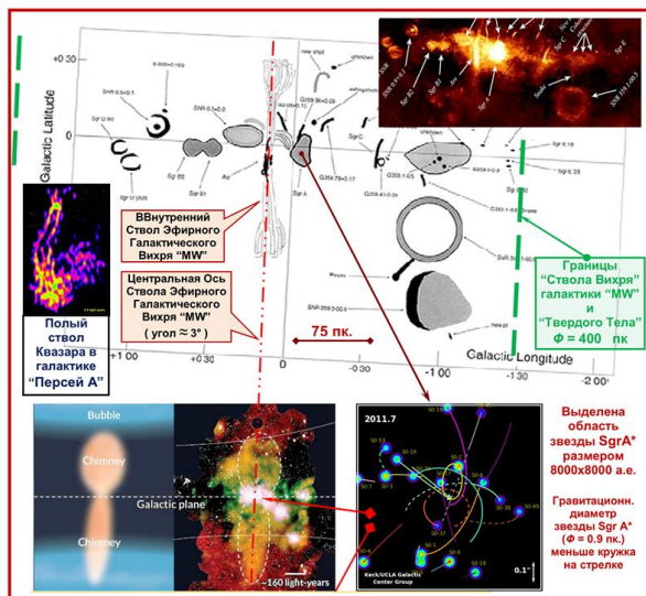
Рис.7. Эфиродинамический двойной Тороидально-Кольцевой вихрь с Джетами Галактики Млечный Путь.
