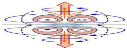
Рис. 6. Эфирный сдвоенный торондальный вихрь звездного или Галактического типа, включая Квазары. Справа схема торонда.
