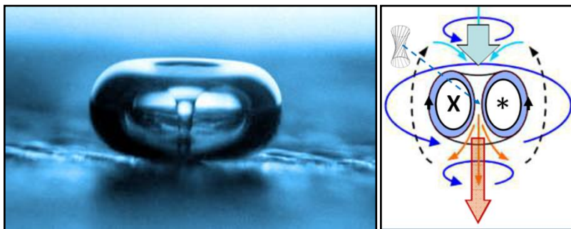
Рис. 17. Crim L. J. Physique, V.40, 285, 1979., КП и Эфиродинамическая модель КП.
