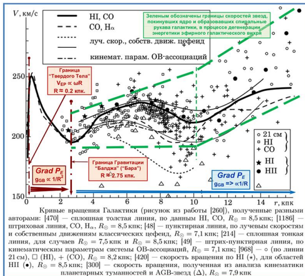
Рис.8. Кривые вращения звезд Галактики Млечный Путь.
