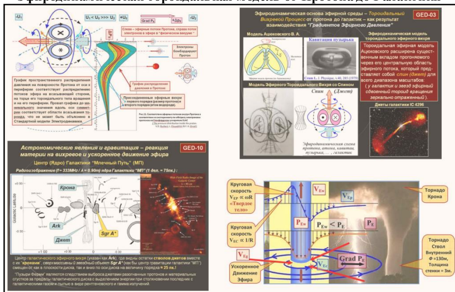
Рис. 0. Обзор приложений эфиродинамической модели к разным физическим процессам.
