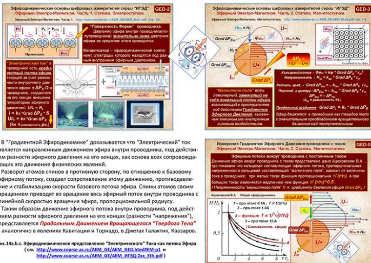
Рис. 14. Эфиродинамическое представление потока эфира в проводнике как “электрического” тока.
