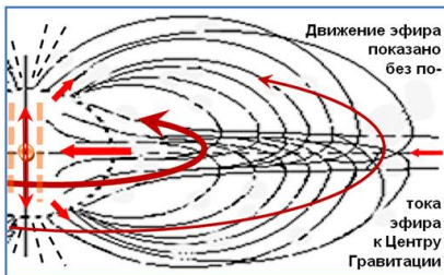
Рис. 6. Эфирный сдвоенный торондальный вихрь звездного или Галактического типа, включая Квазары. Справа схема торонда.
