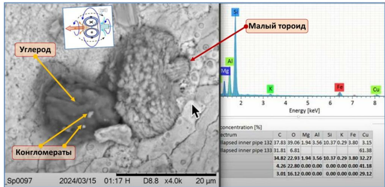
Рис. 21. Выброс углерода кавитационным тороидом и конгломератов с составом, указанным в таблице.
