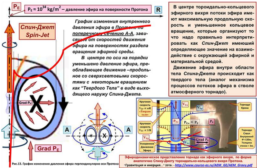
Рис. 13. Изменение эфирного давления перпендикулярно оси через центр Протона.
