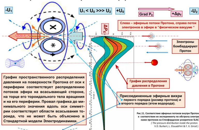
Рис. 11. Соответствие эксперимента SLAC и тороидально-кольцевой со Спино-Джетом.
