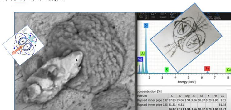
Рис. 19. Спин-Джет тороидальной структуры “кавитационного пузырька” из материалов Р. Гринье.
