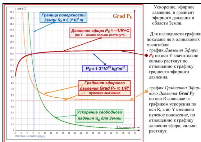
Рис. 9. Графики Эфирного давления, Градиента Эфирного давления, и ускорения в области поверхности Земли внутри нее и за ее пределами. ( Синяя вертикальная черта – это граница поверхности Земли ).
