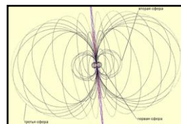
Рис.10. Эфирный Галактический фрактальный вихрь
