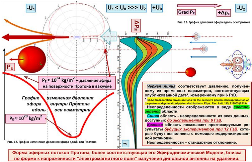
Рис. 12. Изменение эфирного давления вдоль оси Протона.
