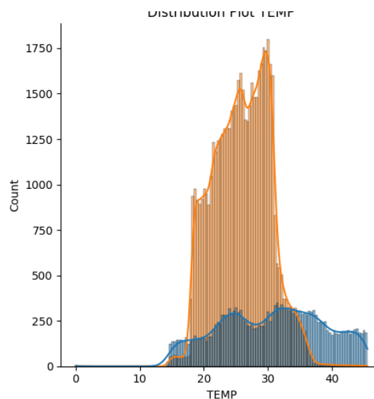
FIGURE 10 – Distribution de la Température selon la qualité de l'eau
