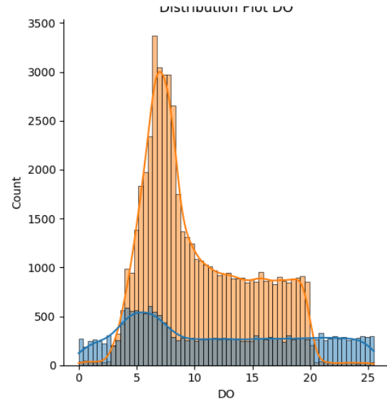
FIGURE 12 – Distribution de l'Oxygène Dissous selon la qualité de l'eau
