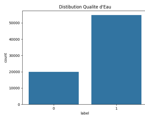
FIGURE 14 – Répartition des classes de qualité de l'eau
