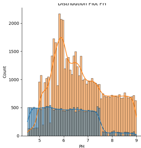
FIGURE 11 – Distribution du pH selon la qualité de l'eau
