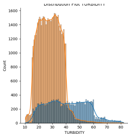
FIGURE 9 – Distribution de la Turbidité selon la qualité de l'eau
