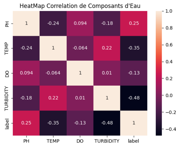
FIGURE 13 – Matrice de corrélation entre les composants de l'eau
