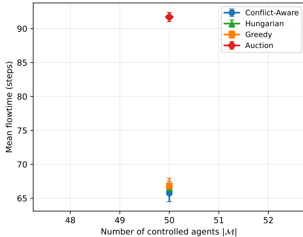
random-64-64-10: Flowtime
