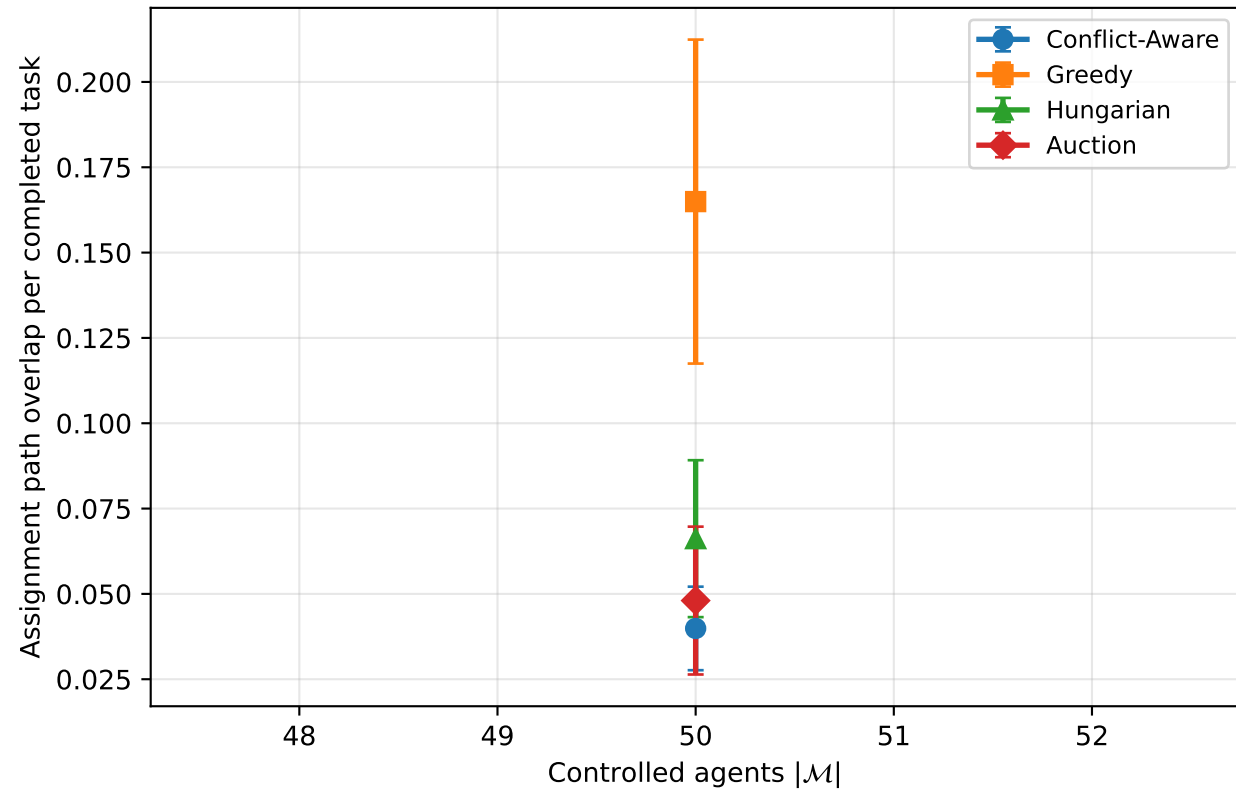
random-64-64-10
