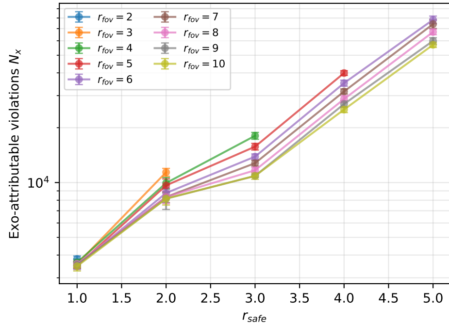
random-64-64-10: N_x vs r_{safe}
