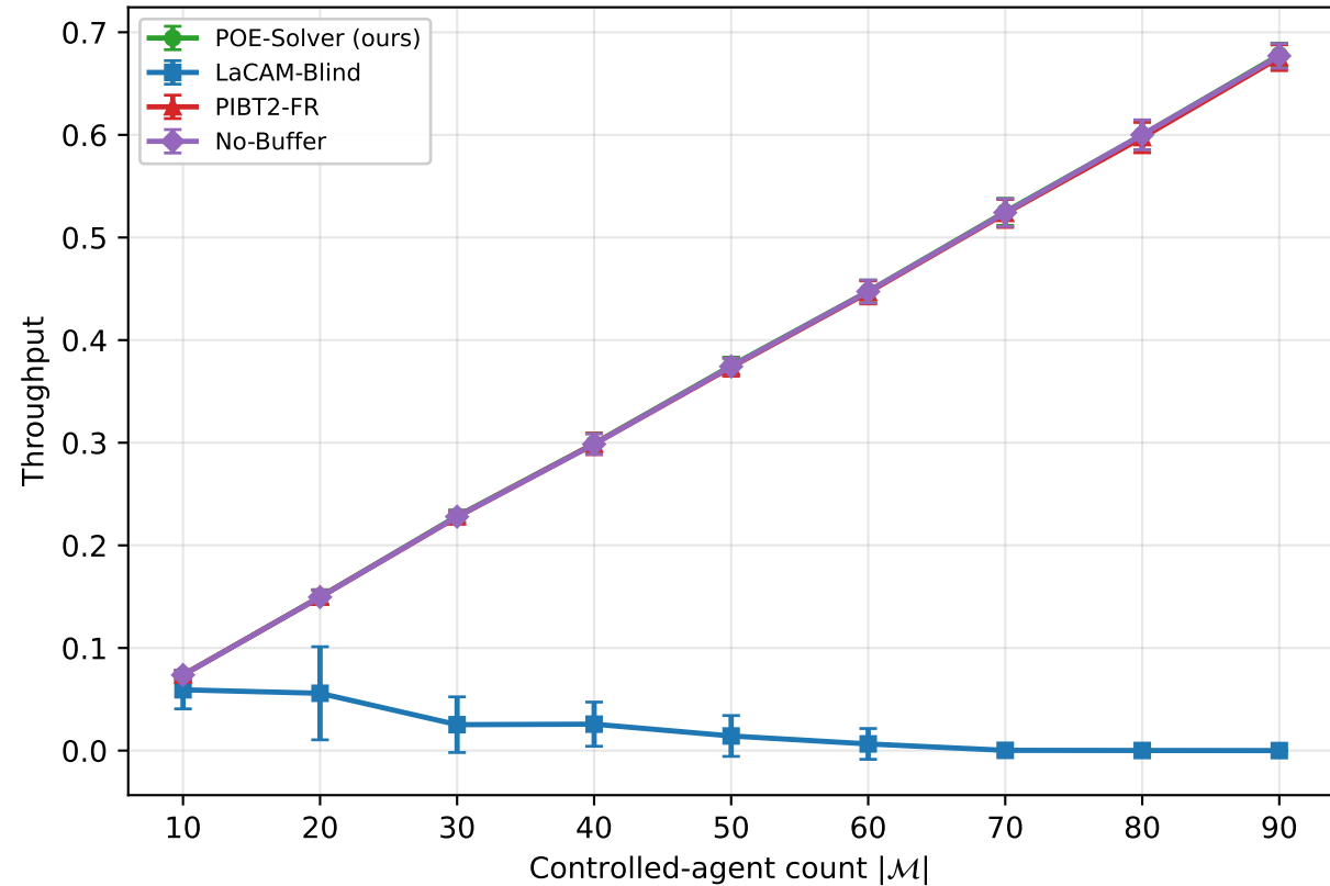
random-64-64-10
