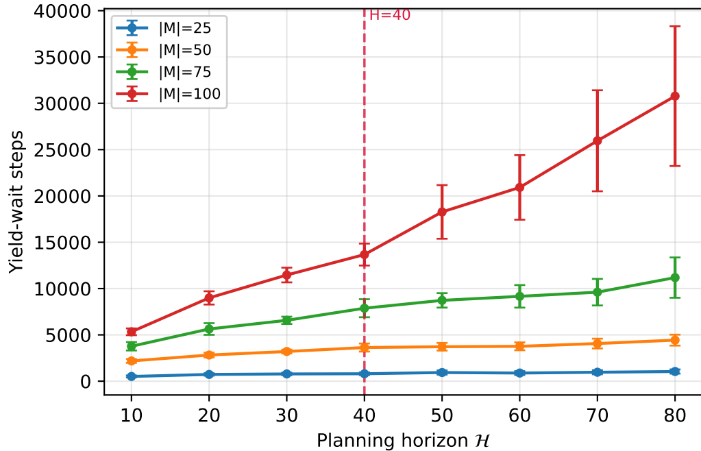
random-64-64-10
