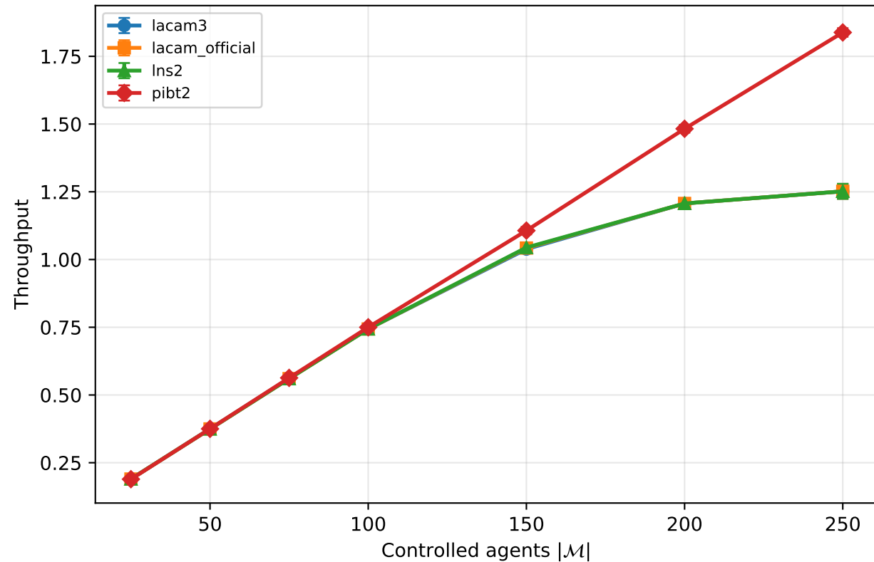
random-64-64-10
