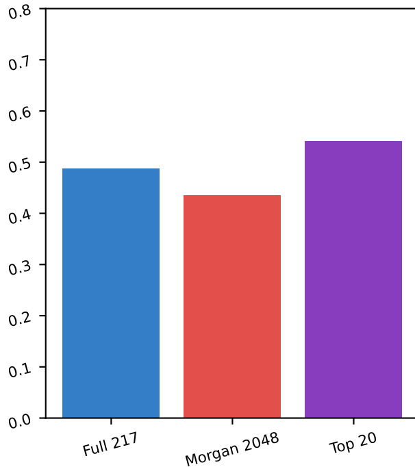
LUMO LOOCV R^2
