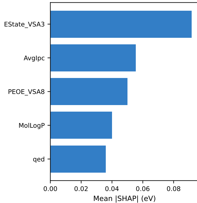
GAP
