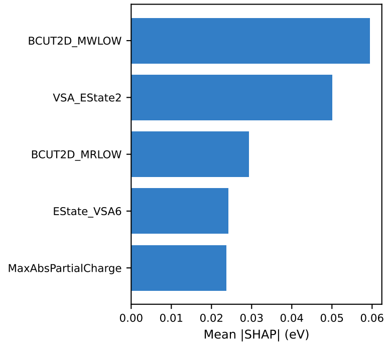
LUMO
