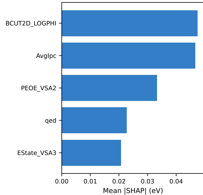
HOMO
