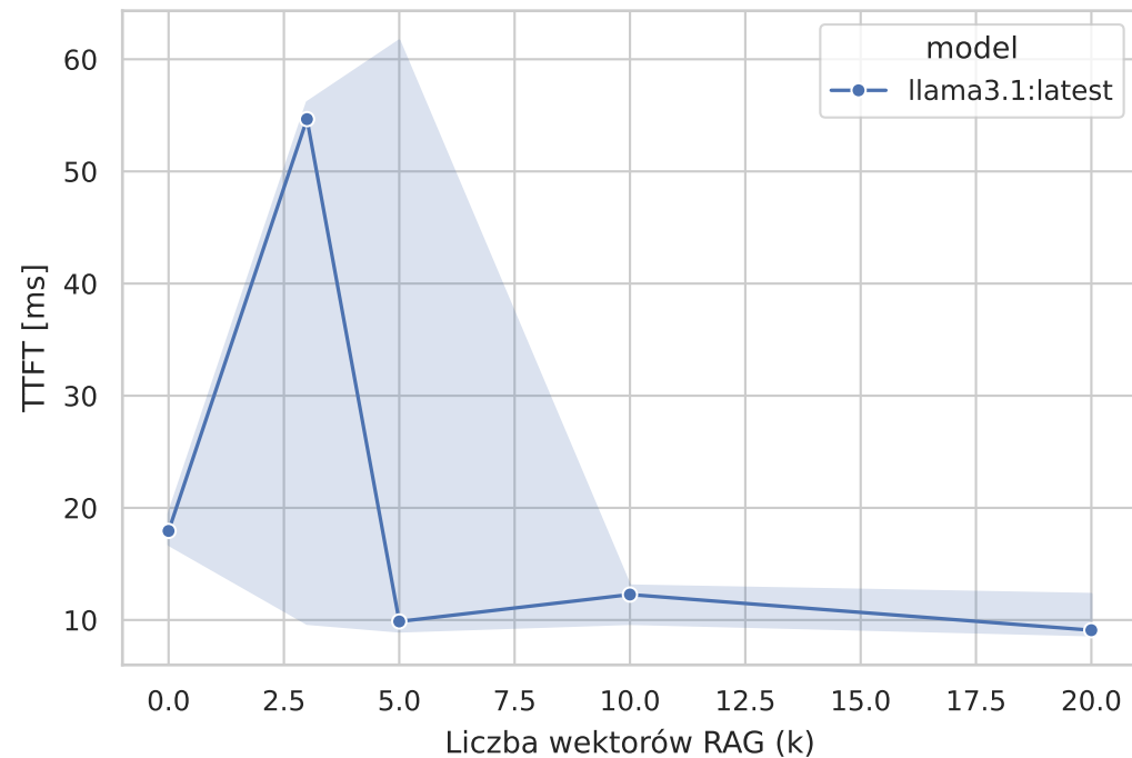
Time To First Token wobec kontekstu RAG
