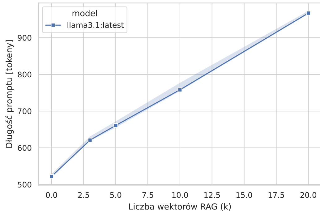
Mechanizm: k -&gt; rozmiar promptu -&gt; czas prefill
