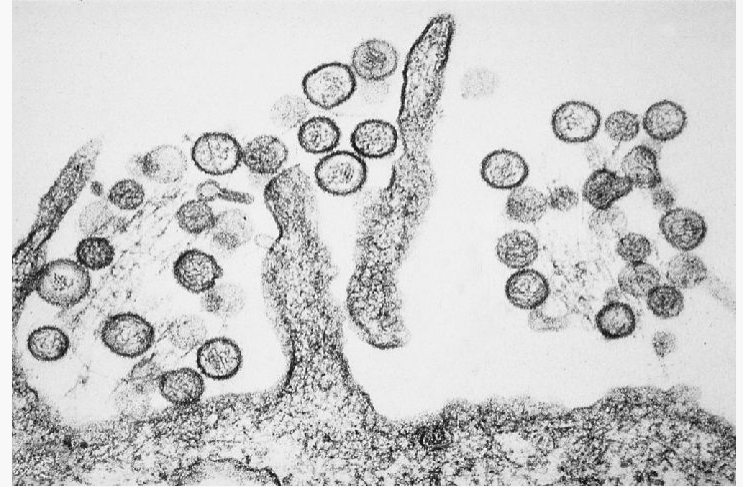
Recuperado de microscopía electrónica de Hantavirus (Centers for Disease Control and Prevention & Goldsmith, Cynthia 1993)
