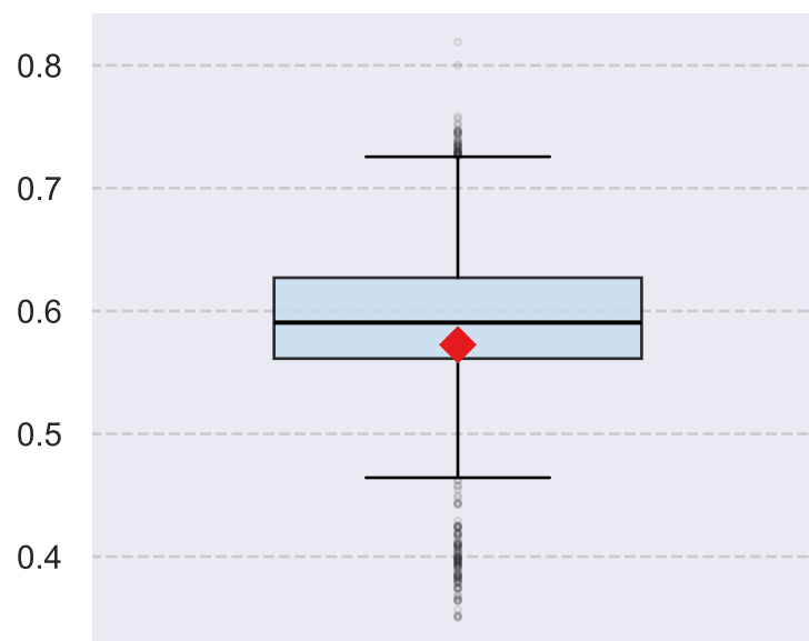
LP spikes/burst
