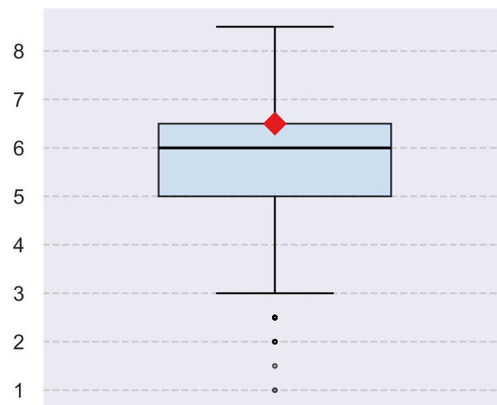
LP spikes/burst
