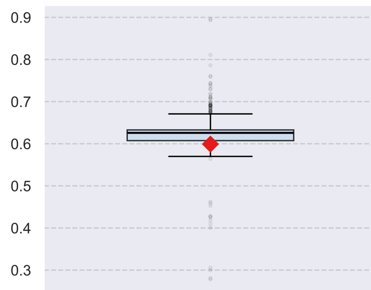
PY spikes/burst
