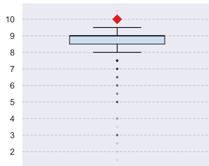
PY spikes/burst
