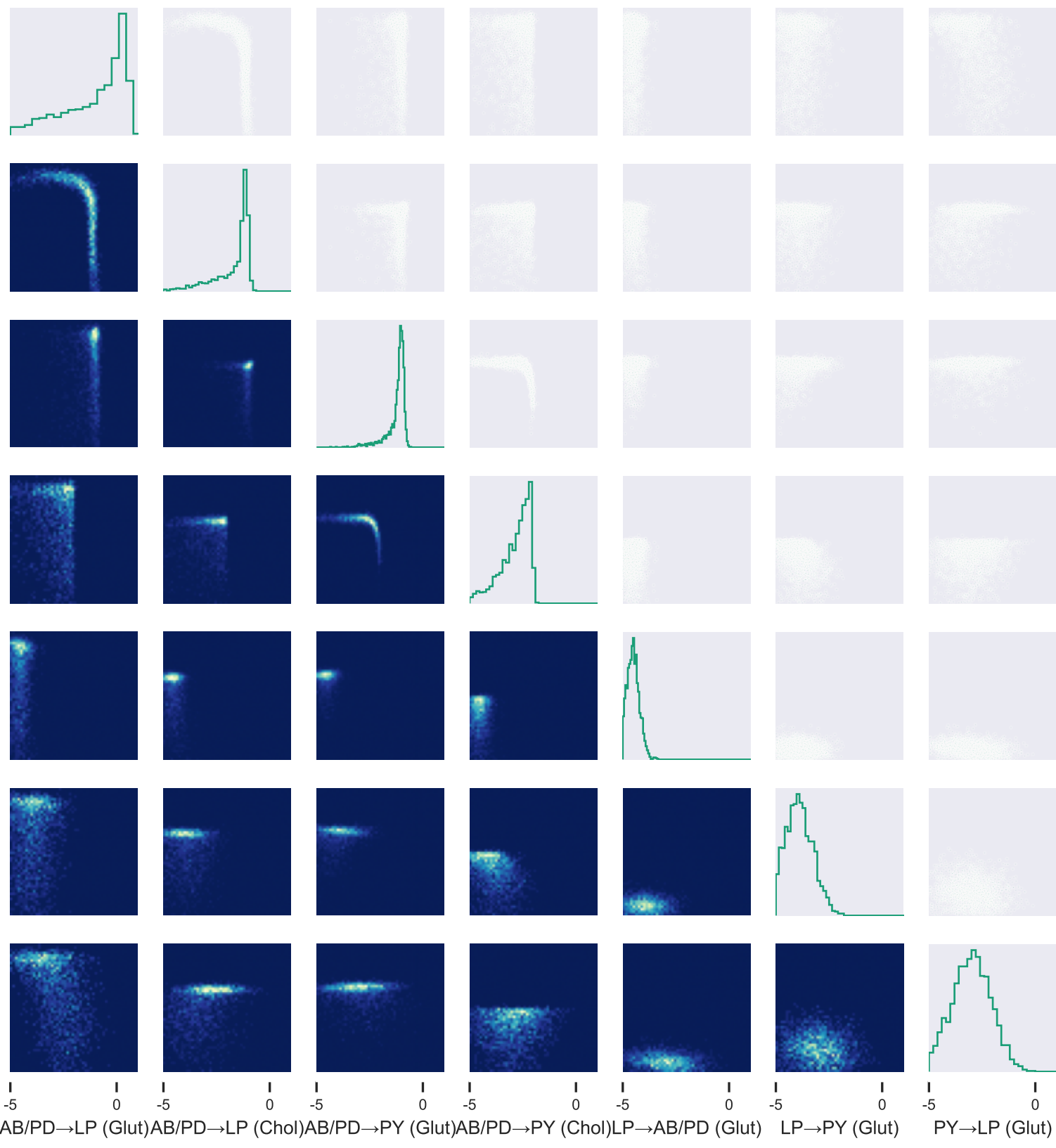
SNPE posterior — \log_{10}(g_{\text{syn}} / \mu\text{S})
