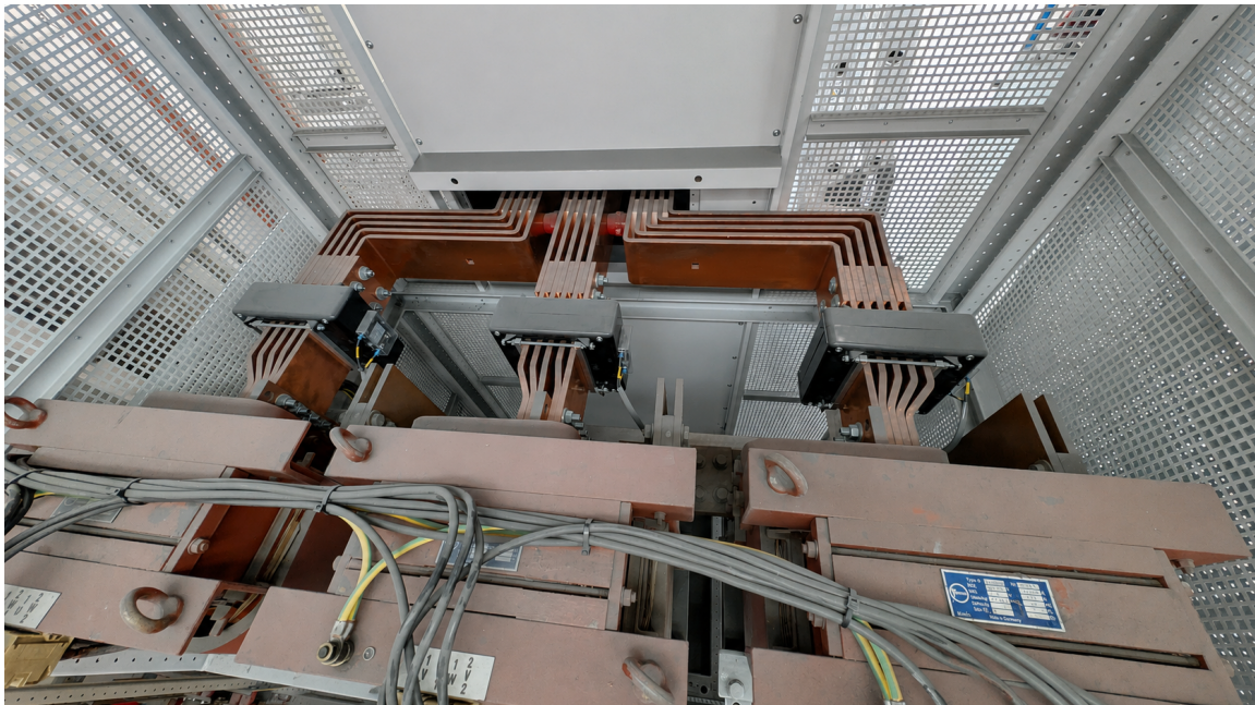
Abbildung 3.5: Festtransformator mit sekundärseitigen Hochstromverbindungen und den drei nachgeschalteten Stromwandlern (eigene Aufnahme)
