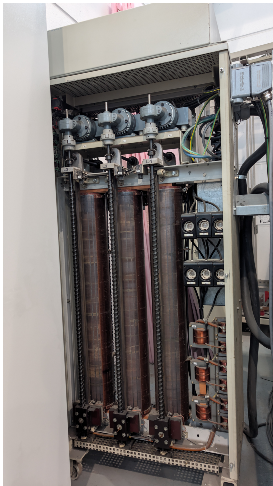
(a) Stelltrafo
