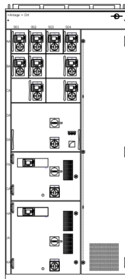
Abbildung 2.2: Frontansicht des MCC-Feldes bestückt mit Einschubmodulen
