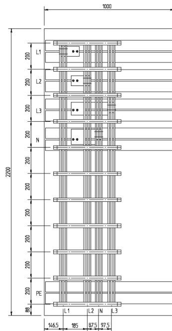
Abbildung 2.3: Vertikales Verteilschienensystem
