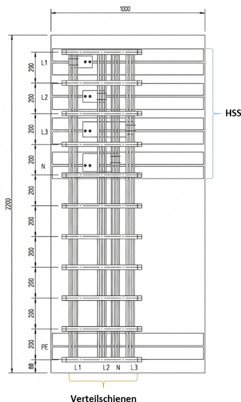
Abbildung 2.4: Vertikales Verteilschienensystem
