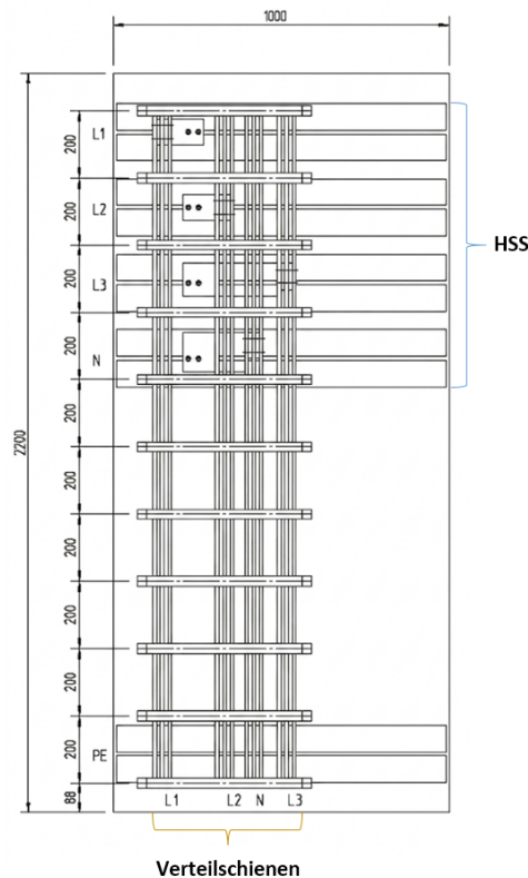
Abbildung 3.4: Vertikales Verteilschienensystem
