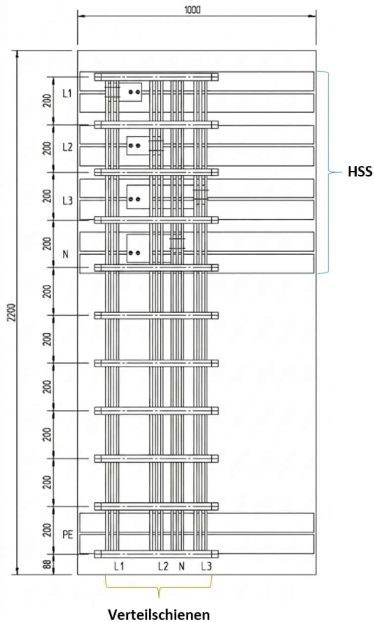
Abbildung 2.4: Vertikales Verteilschienensystem
