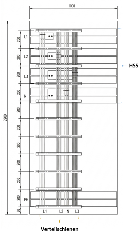
Abbildung 3.4: Vertikales Verteilschienensystem
