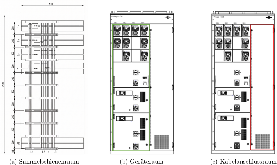
Abbildung 7.3: innerer Unterteilung des MCC-Feldes
