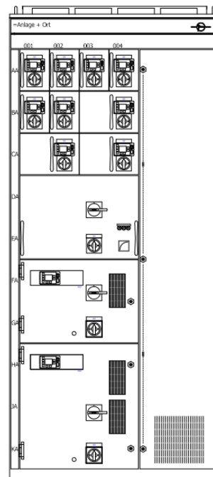
Abbildung 7.2: MCC-Feld bestückt mit Einschubmodulen
