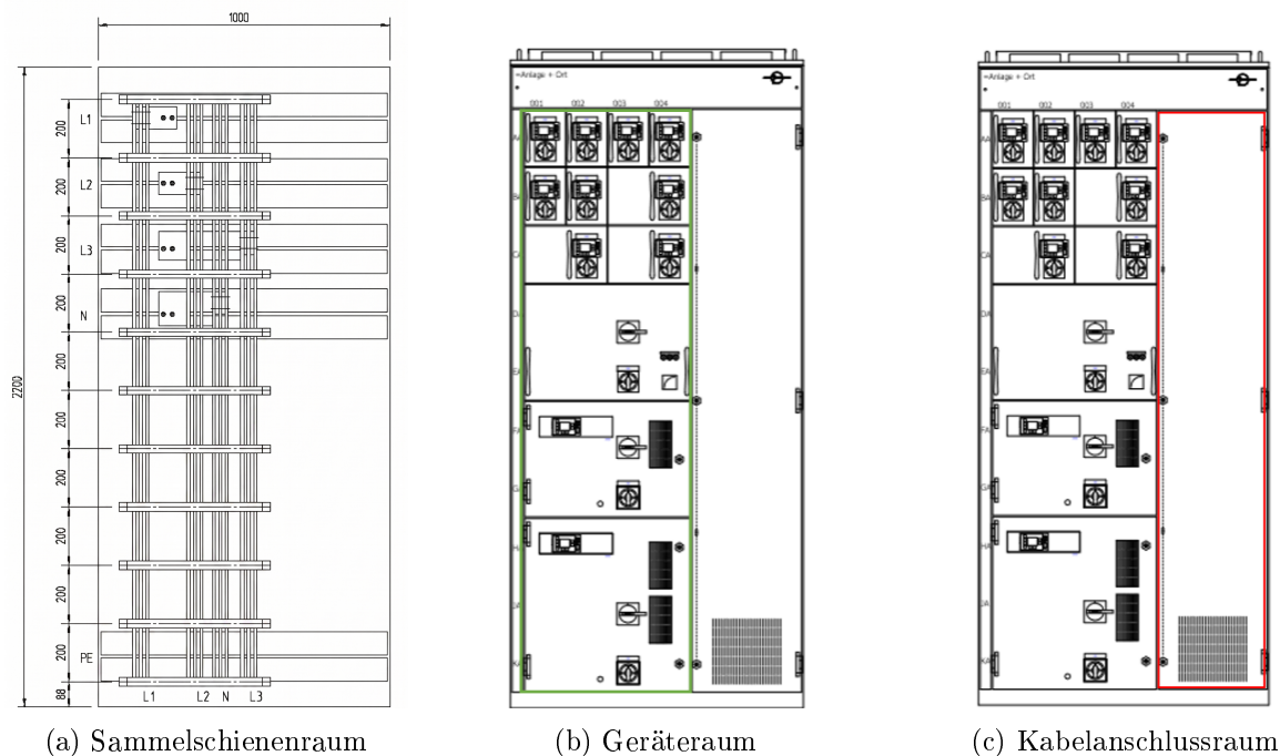
Abbildung 6.3: Funktionsbereiche des MCC-Feldes
