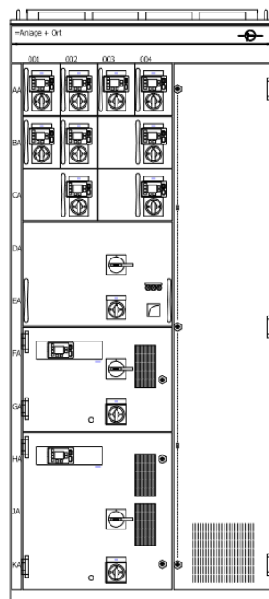
Abbildung 6.2: MCC-Feld bestückt mit Einschubmodulen
