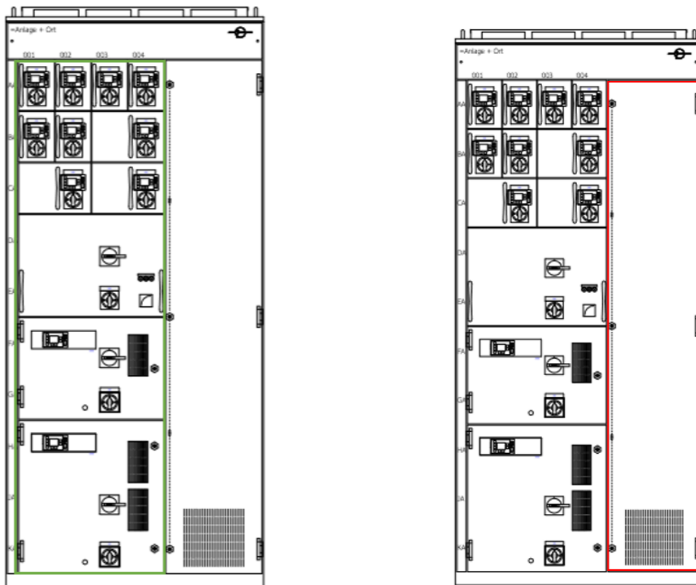
Abbildung 3.8: Kennzeichnung des Geräteraums (links) und des Kabelanschlussraums (rechts) am betrachteten MCC-Feld (betriebsinterne Darstellungen)
