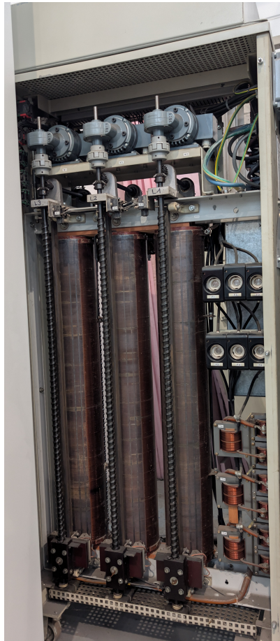
Abbildung 3.3: Geöffneter Säulenstelltransformator mit drei Wicklungssäulen, sechs Stromabnehmern und drei motorischen Antrieben (eigene Aufnahme)
