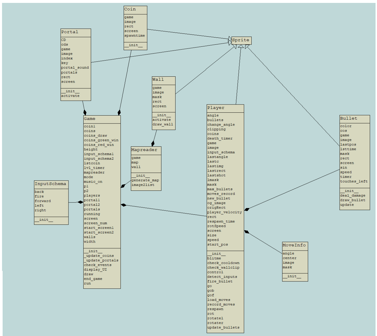
Рис. 1: UML диаграмма
