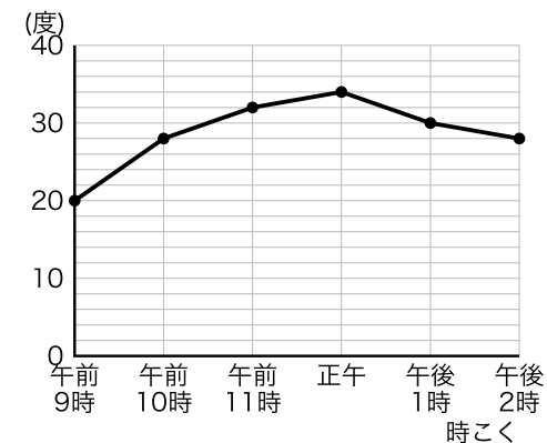
すな場のすなの温度
