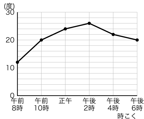
池の水温
