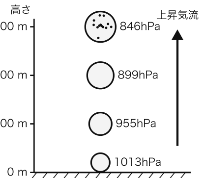
上昇する空気と雲
