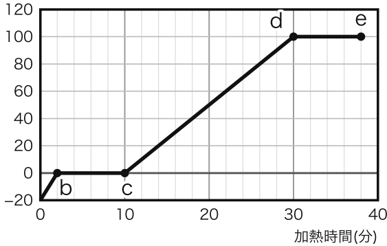
図2 液体Xを一定の火力で加熱 温度(℃)
