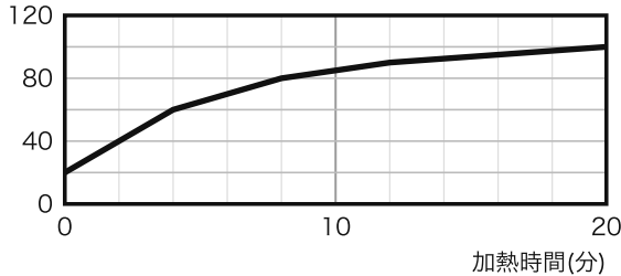
図2 液体Xを一定の火力で加熱 温度(℃)
