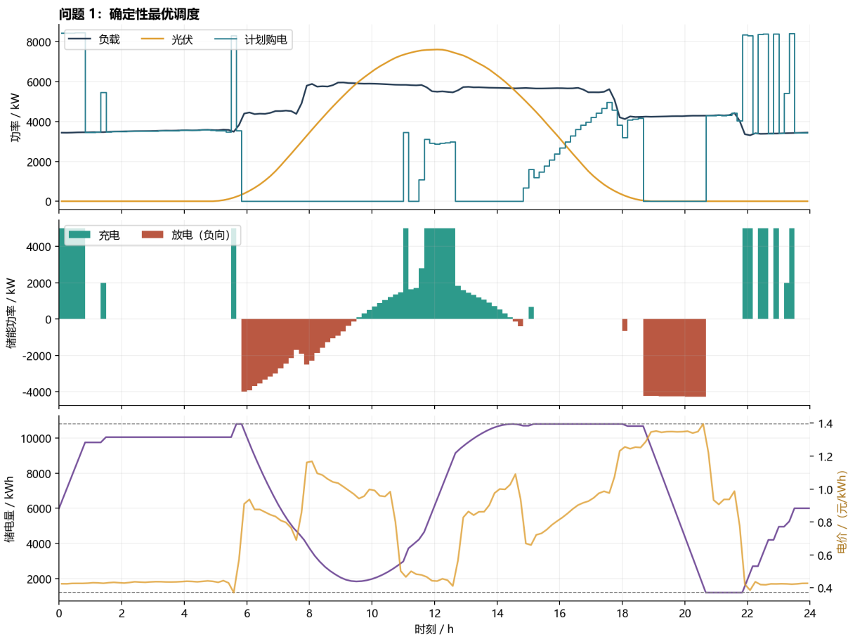
图 1 问题一的最优购电与储能调度
