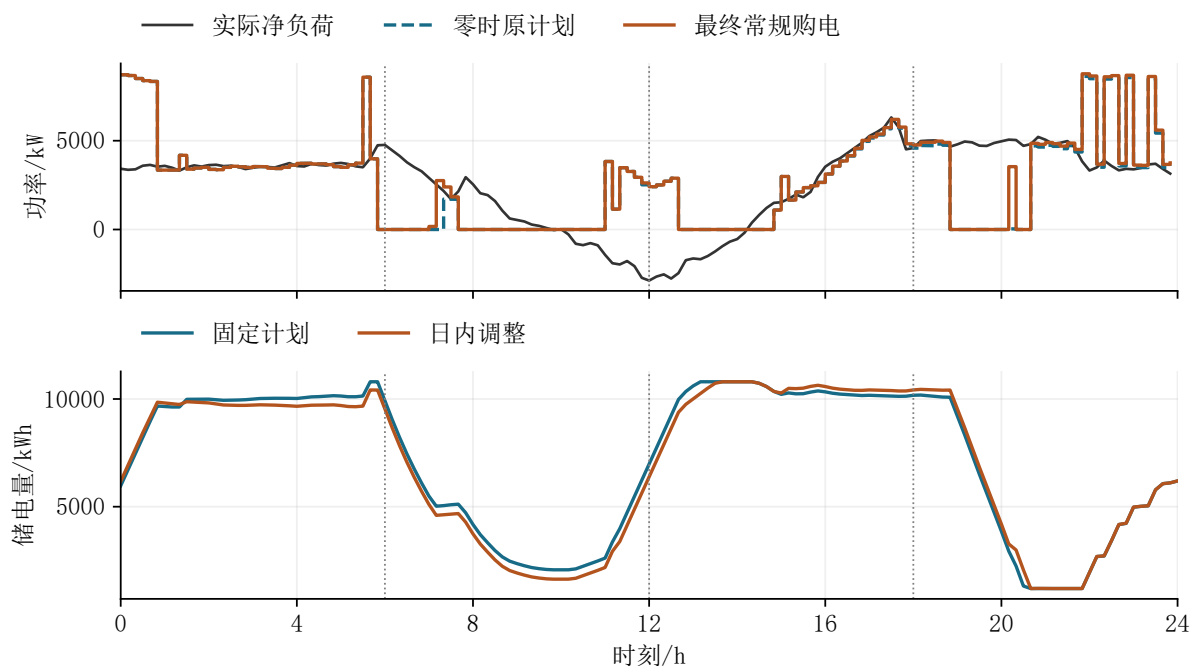
图3 9月23日的日内购电调整与库存变化
