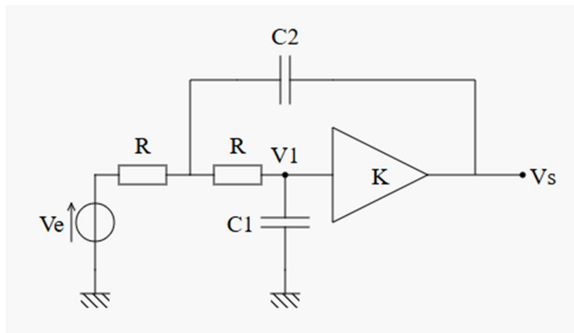
Figure 11 Montage Filtre Sallen-Key d'ordre 2
