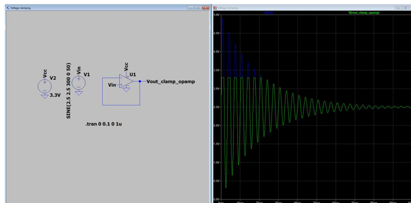
Figure 8 Circuit de clantage entrée analogique avec AOP
