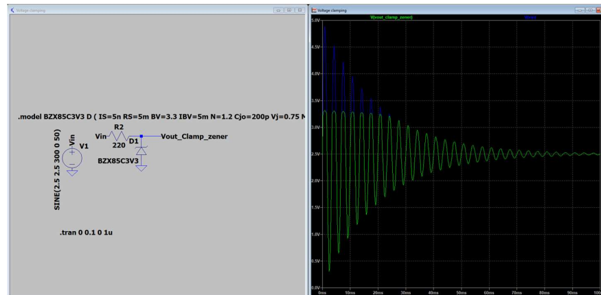
Figure 7 Circuit de clantage entrée analogique avec diode Zener
