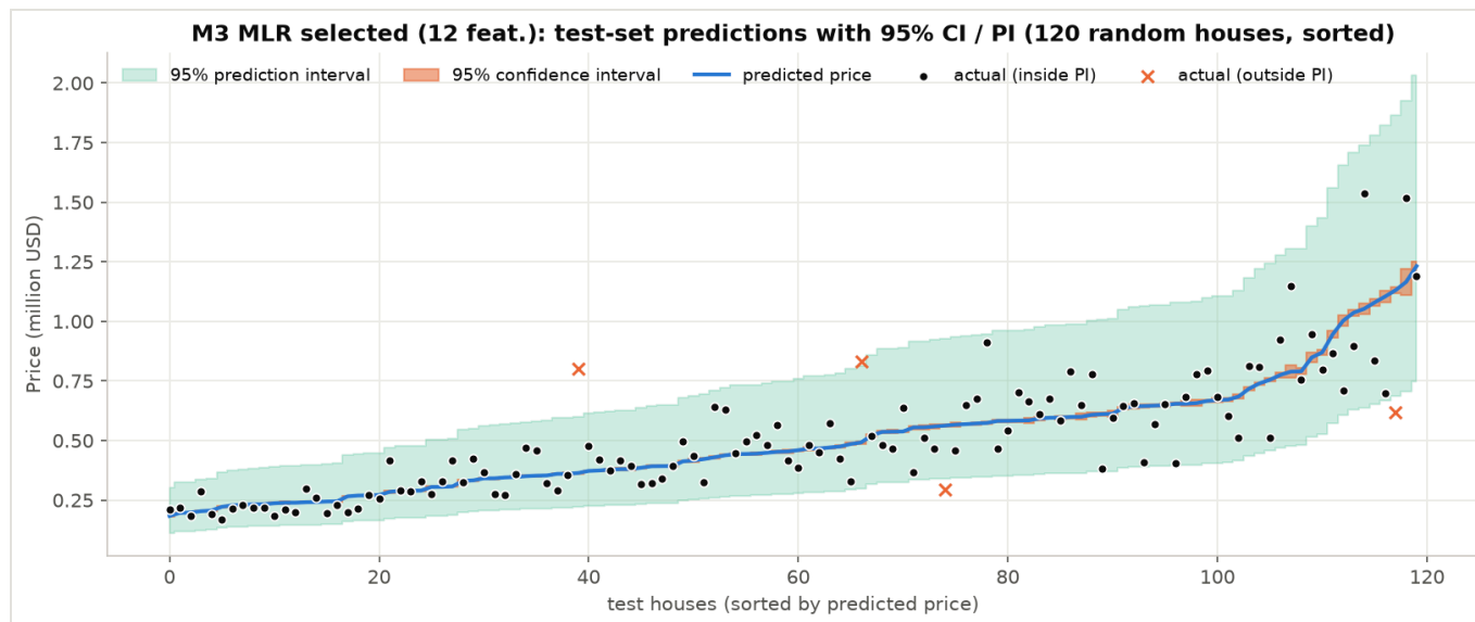
圖 9 M3 預測圖：隨機 120 間測試房屋，依預測值排序；× 為落在 95% PI 外的房屋
