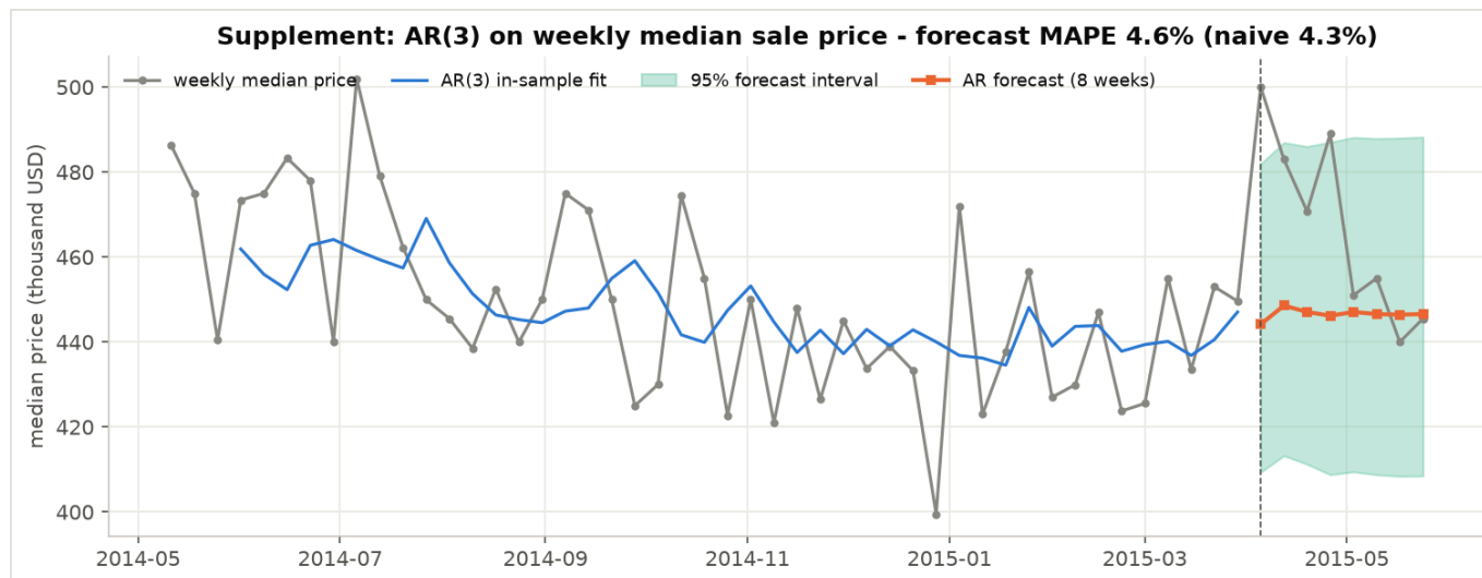
圖 7 AR(3) 預測每週中位房價：MAPE 4.6%，比「直接沿用上週值」的 naive 預測（4.3%）還差；95% 預測區間只涵蓋 8 週中的 6 週（75%）
