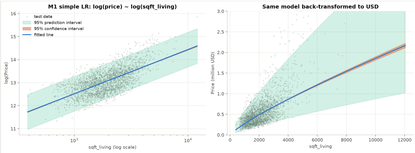
圖 8 M1 單純線性回歸：擬合線、95% 信賴區間 ( 橘，平均價格的不確定性 ) 與 95% 預測區間 ( 綠，單一房屋的不確定性 )
