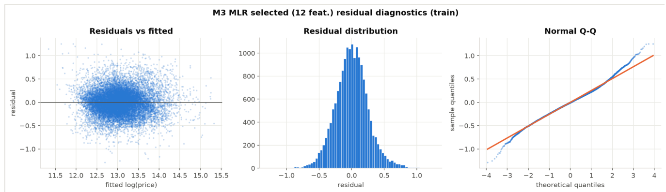
圖 12 M3 殘差診斷：殘差無明顯趨勢、近似常態 ( 尾部略厚，峰度 4.0 )
