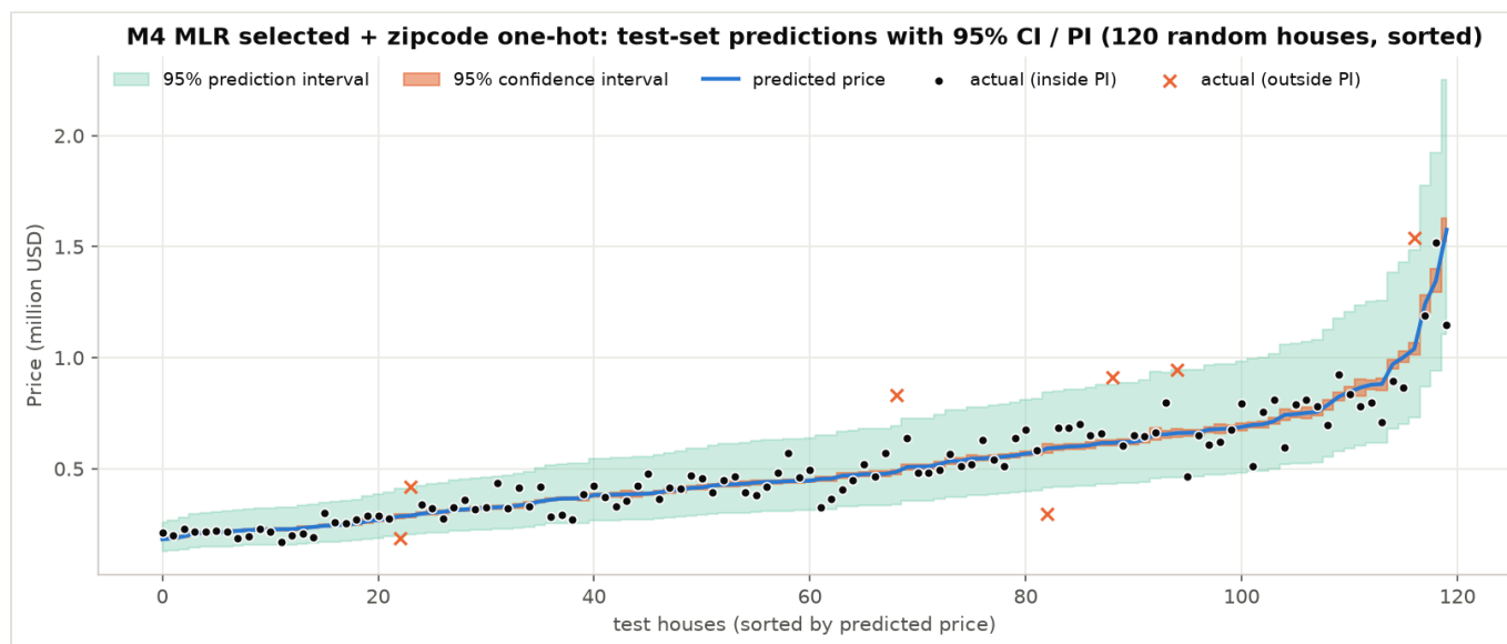
圖 10 M4 (加 zipcode) 預測圖：預測區間明顯變窄 (中位寬度 $474K → $330K)
