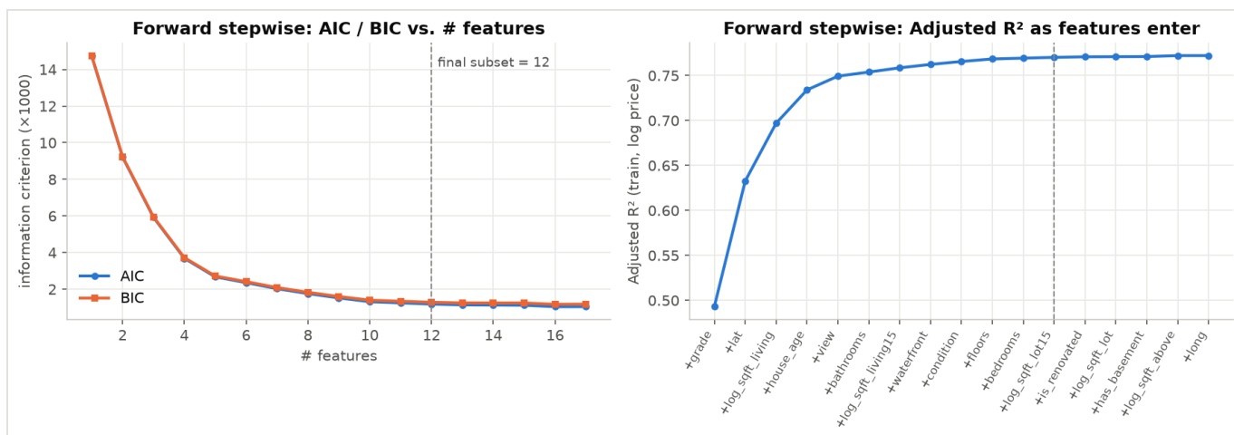
圖 5 Forward Stepwise：左為 AIC/BIC，右為 Adjusted R 2 隨特徵加入的變化。12 個特徵之後曲線已經平了
