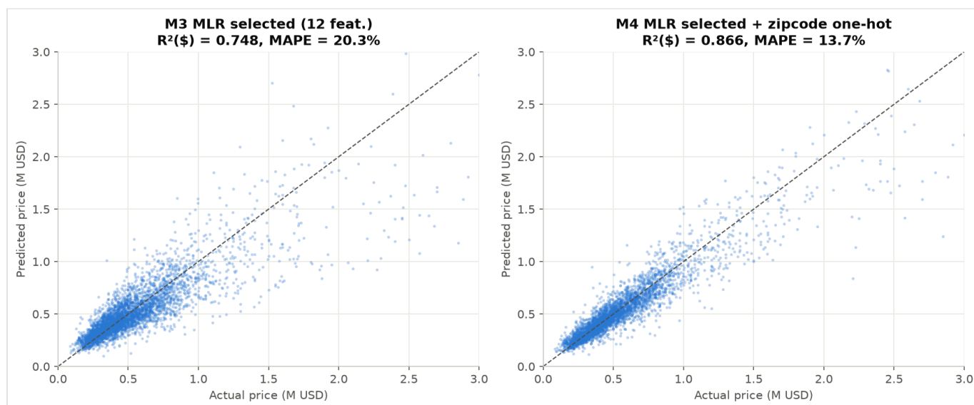
圖 11 實際 vs 預測 (虛線為完美預測)
