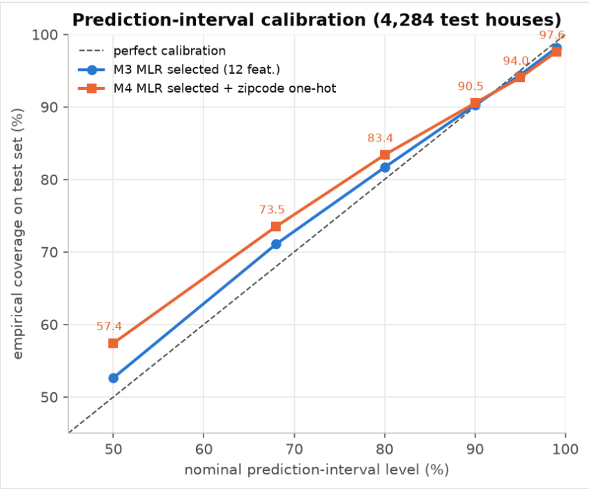
圖 14 預測區間校準圖：越接近虛線越準。90–95% 幾乎完全吻合；低水準時略為保守、99% 略不足，這和殘差「中間尖、尾部厚」( 峰度 4.0 ) 一致
