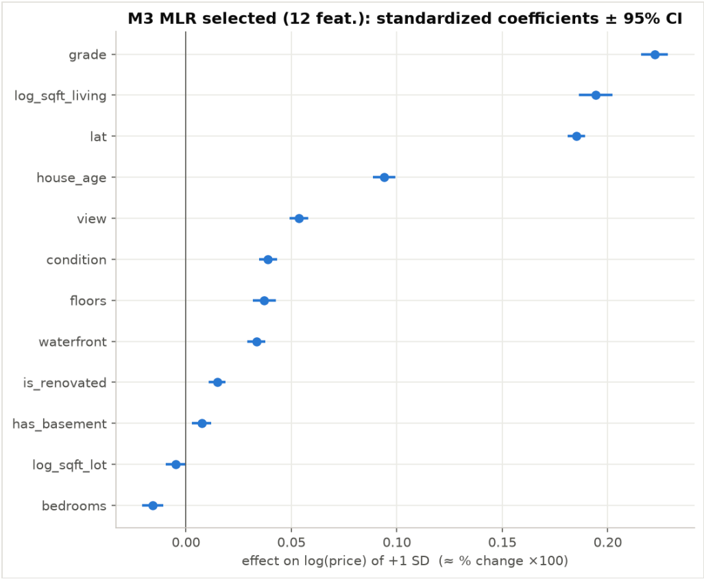
圖 6 M3 標準化係數與 95% 信賴區間 ( 所有區間皆不跨 0 )
