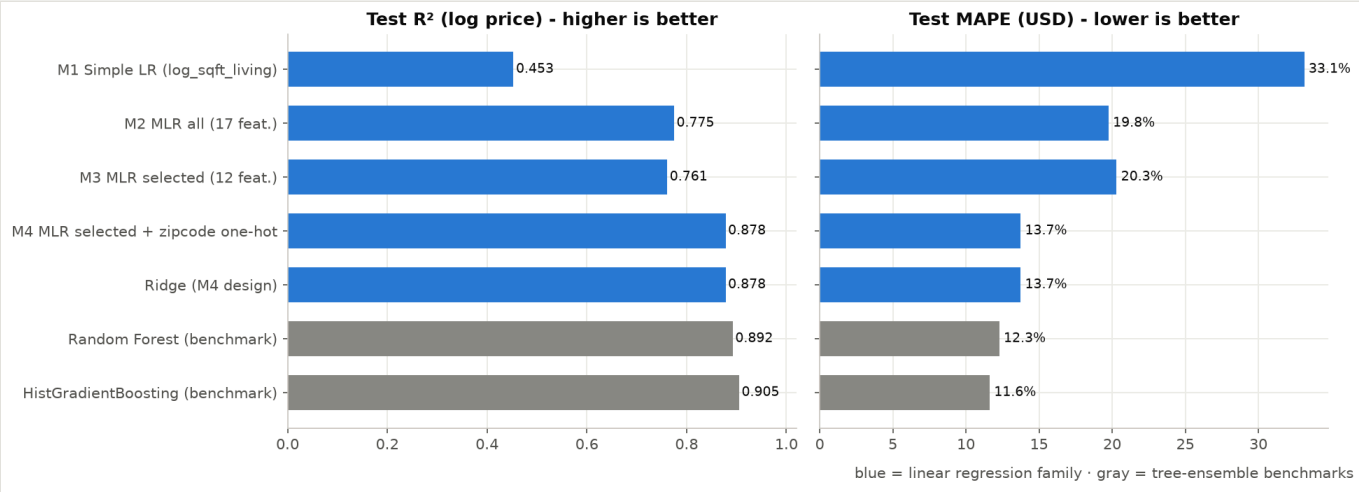
圖 15 模型比較 ( 藍 = 線性回歸家族，灰 = 樹模型對照 )
