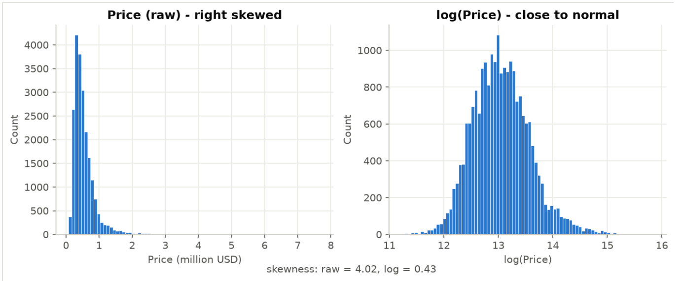
圖1 價格分佈：原始值右偏，取 log 後接近常態
