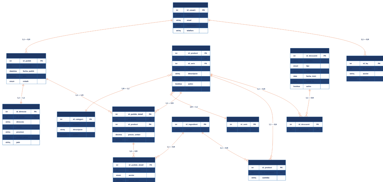
Figura: Diagrama entitat-relació de Crunchyroll Eats: taules, atributs, claus primàries i foranes, i cardinalitats de les relacions entre entitats.
