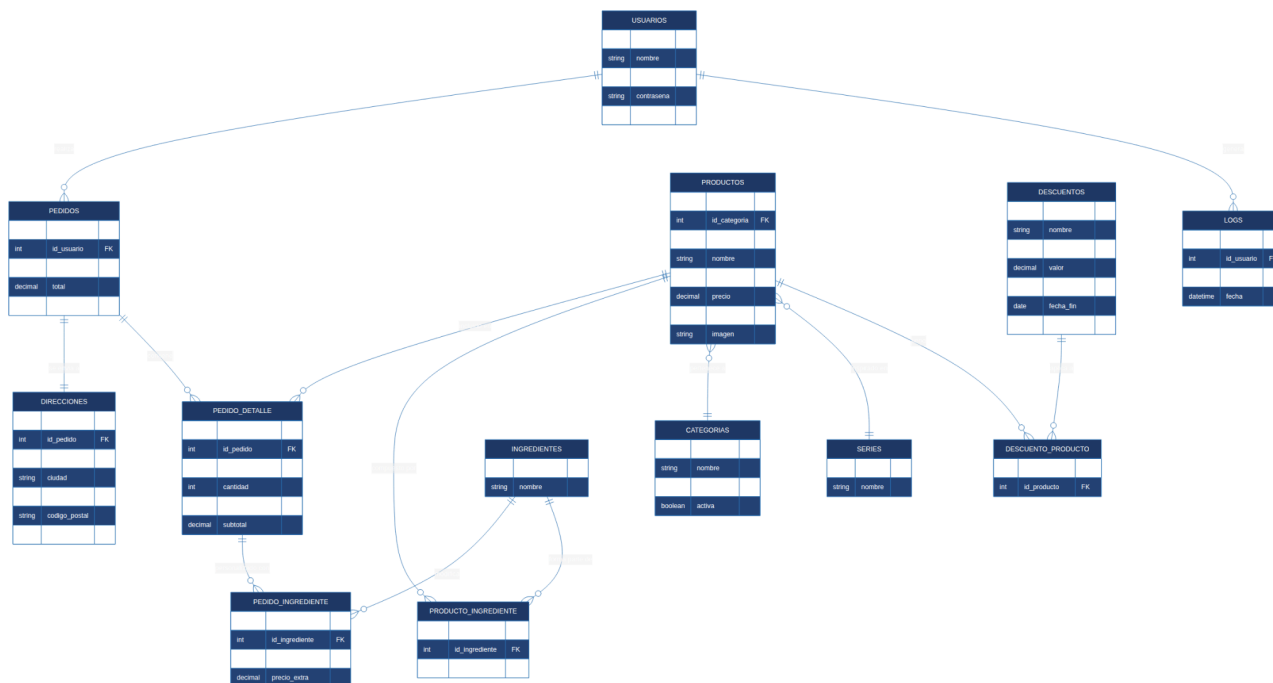
Figura: Model relacional de Crunchyroll Eats: representació de les taules, claus foranes i connexions entre entitats que defineixen l'estructura de la base de dades
