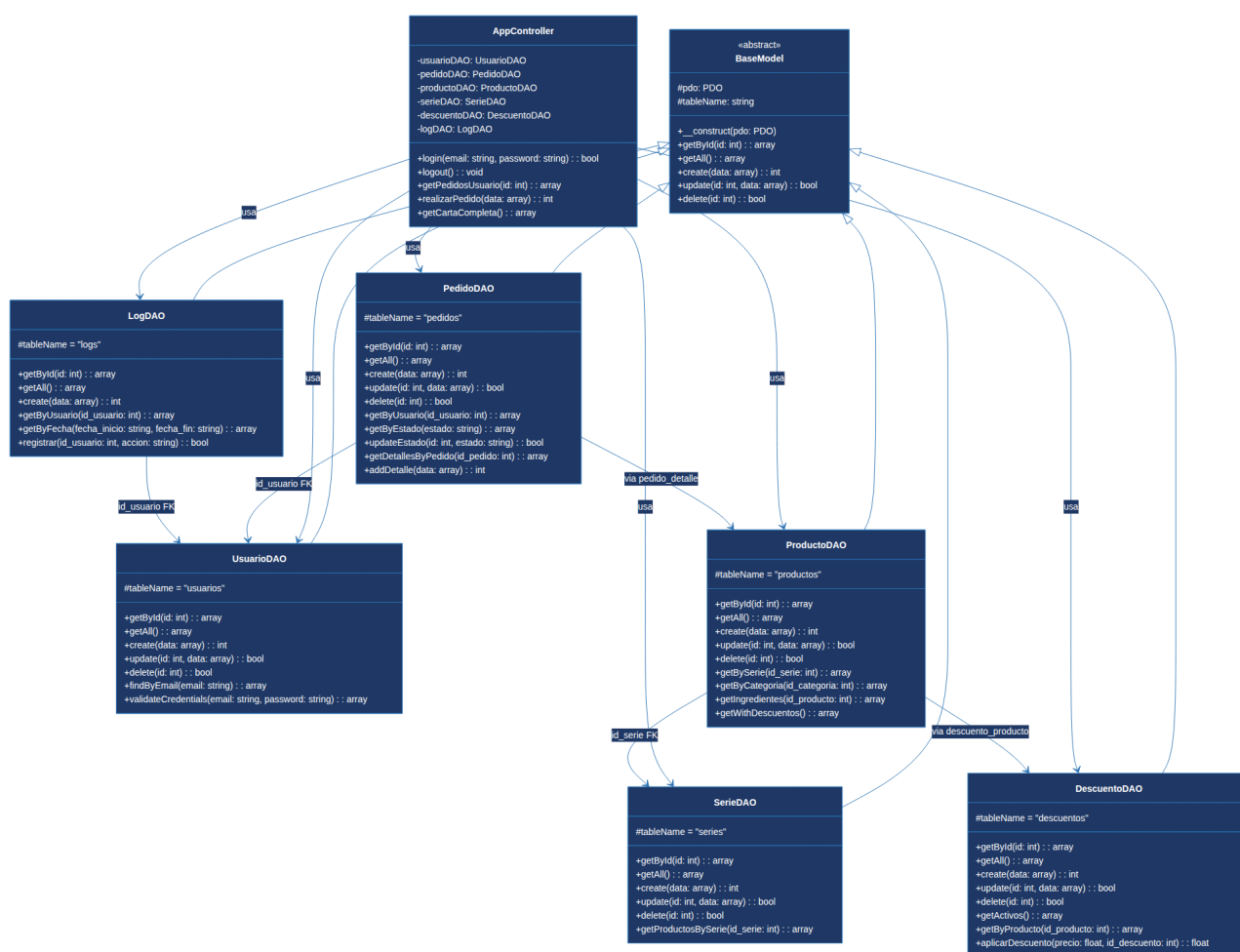
Figura: Diagrama de classes de Crunchyroll Eats: jerarquia d'herència des de BaseModel, classes DAO per entitat, AppController i relacions entre capes de la arquitectura MVC.
