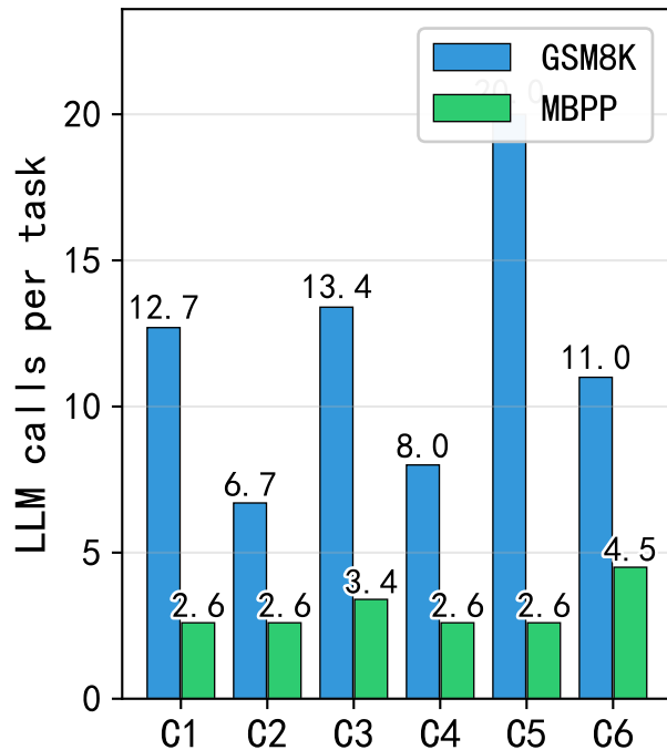
LLM Calls per Task
