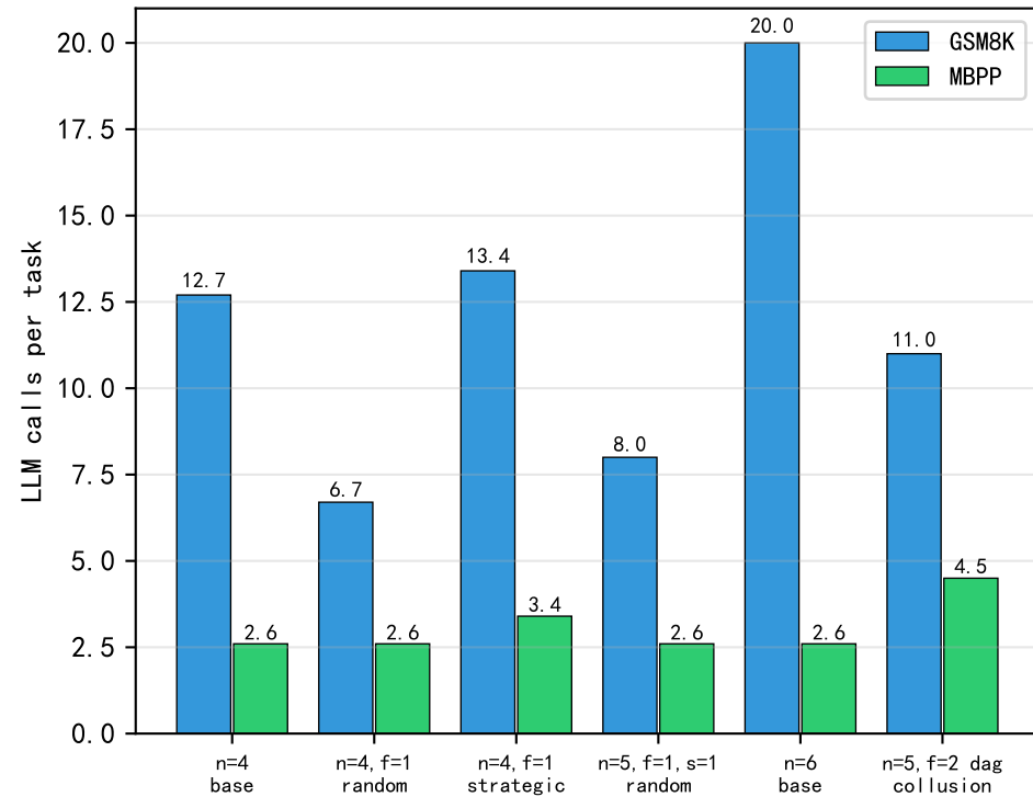
LLM Calls per Task
