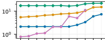
POTRF
