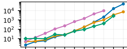
POSV
