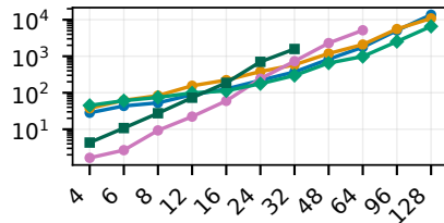
POSV
