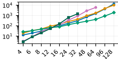
POTRF
