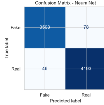
(d) Neural Network Confusion Matrix
